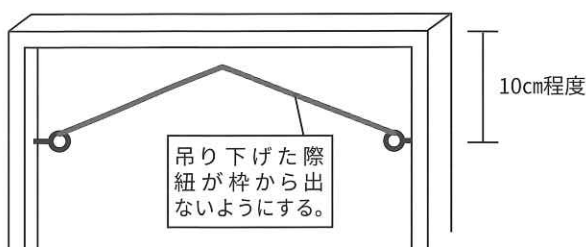
写真作品ヒートンおよび紐取付け図(例)
