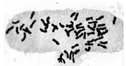
写真2 ノジギク (2n=54) の染色体
