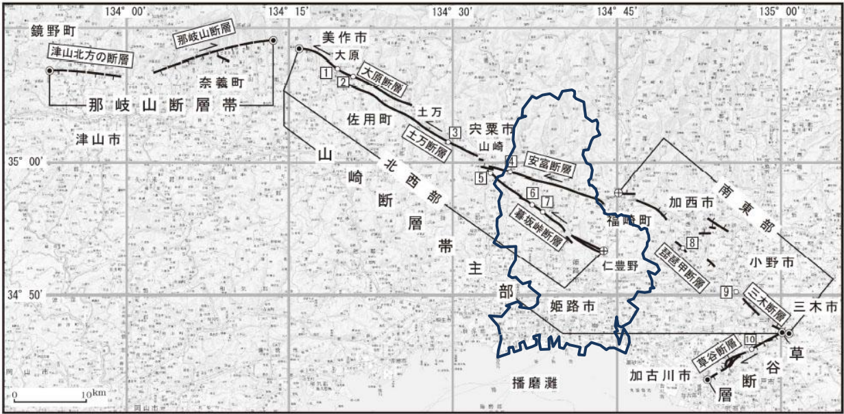
(参考) 地震調査研究推進本部地震調査委員会の長期評価(山崎断層帯主部の評価)
