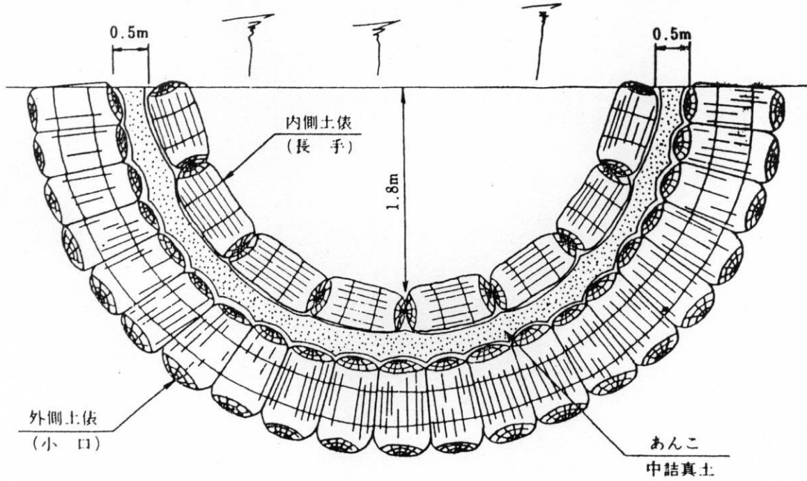
平面図 (第1段)
