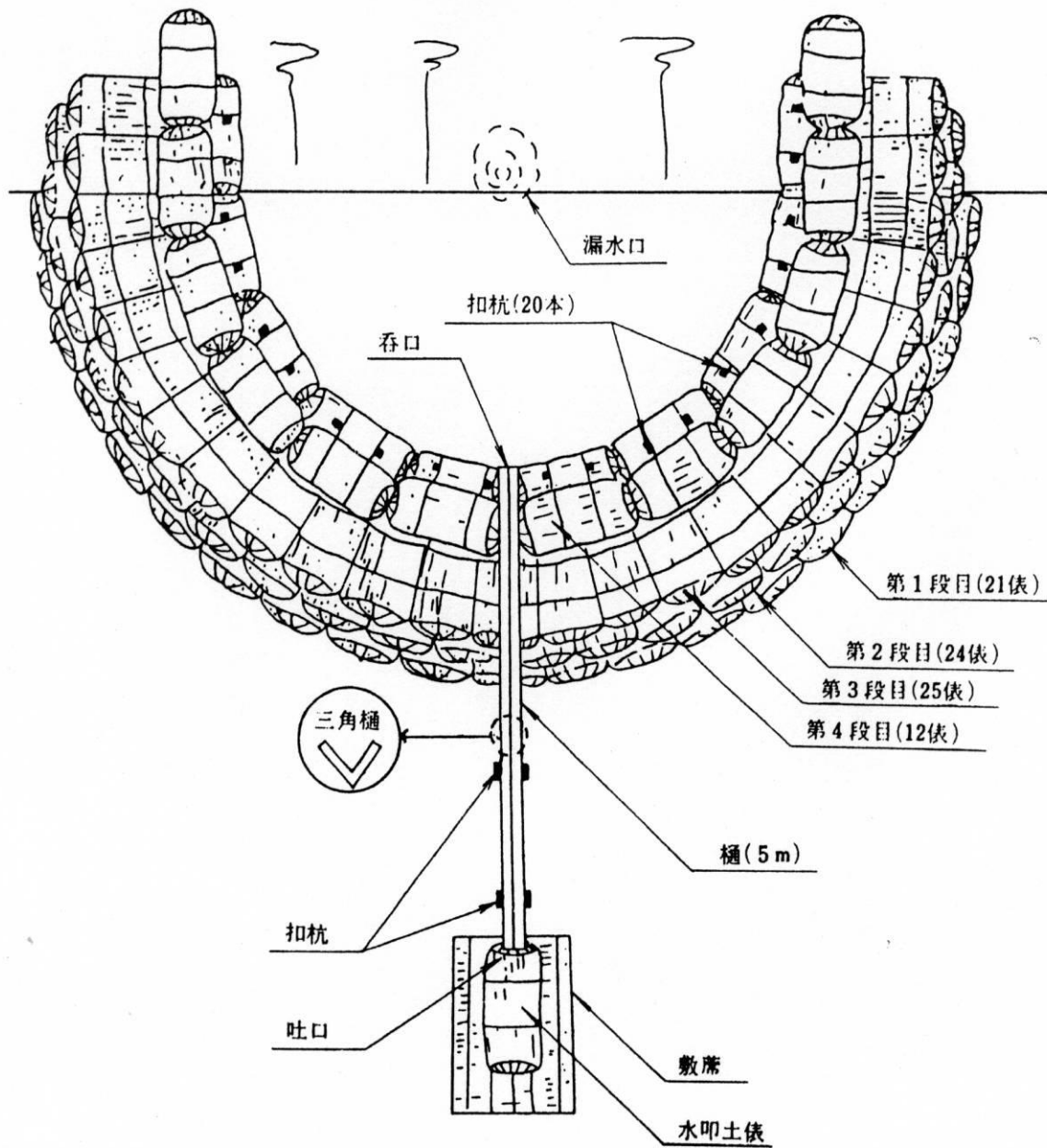
平面图 (完成)
