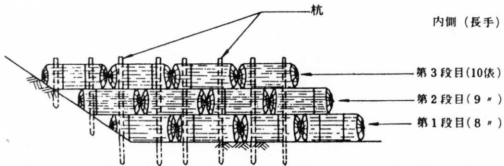
外面断面図
