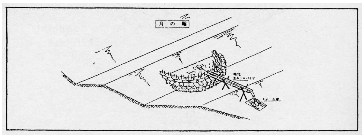
月の輪数量表〔土のう使用〕（１ヶ所当り＝半径1.5m）
