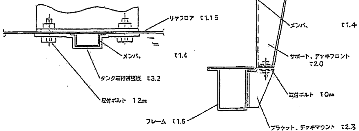
① 部詳細
