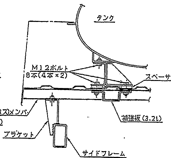
D-D 断面図
