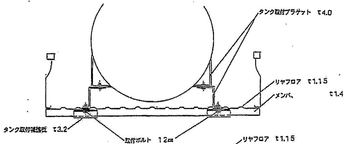
断面A-A矢視図
