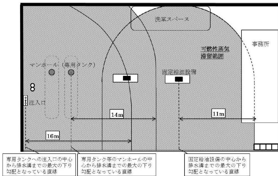
図4 給油取扱所(平面図)
