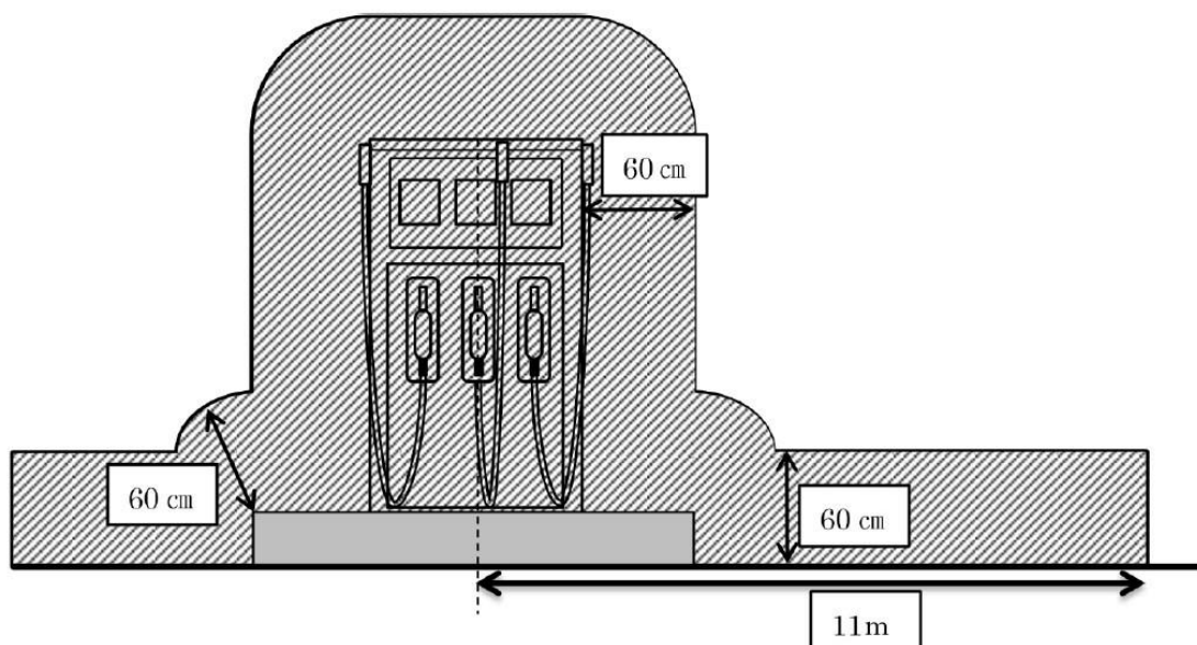
図1 固定給油設備の周囲
