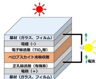
図2 ペロブスカイト太陽電池の構造例 b
