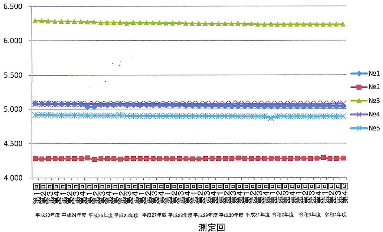
図 1 - 4 地盤沈下推移
