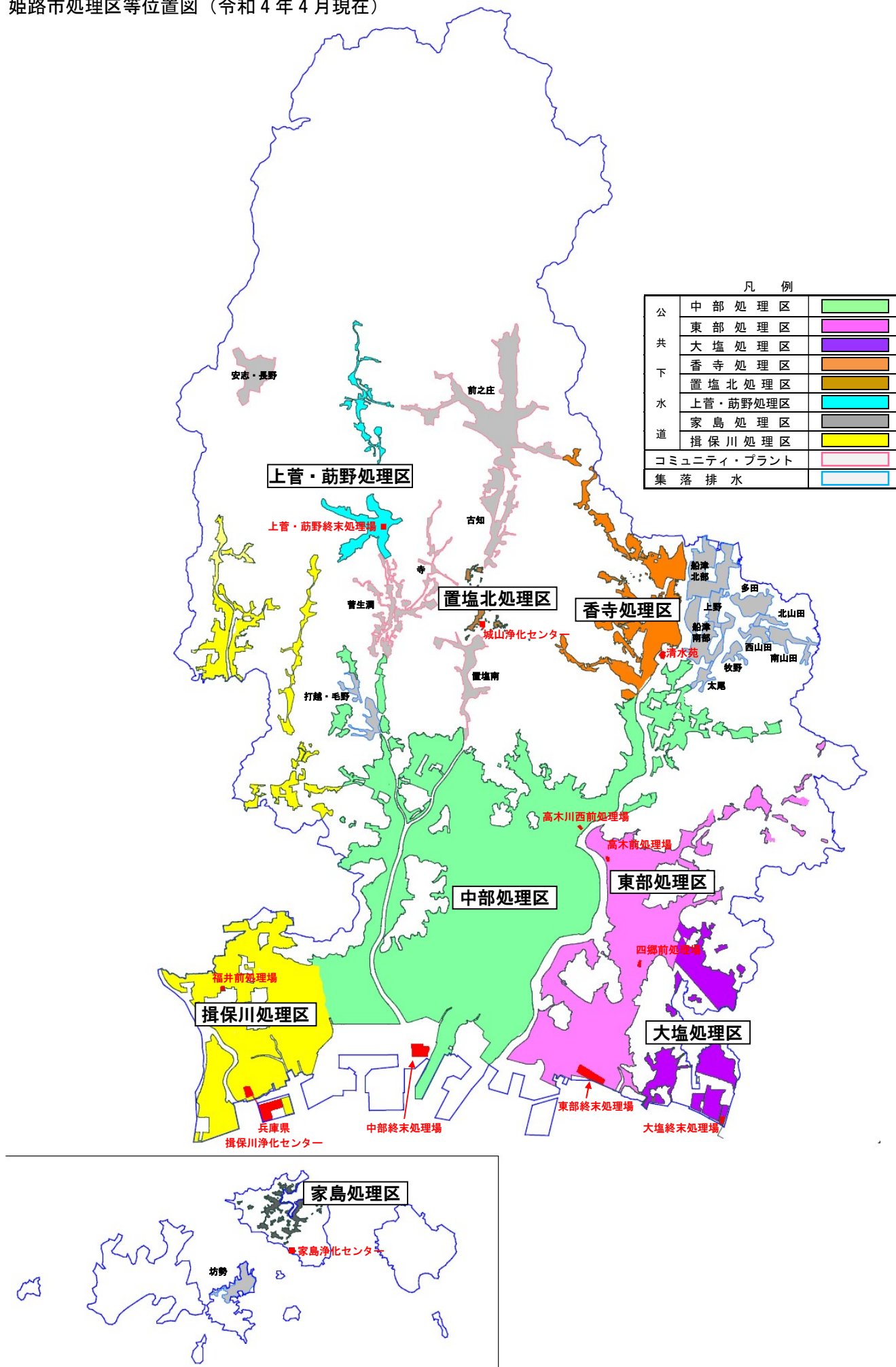
図 姫路市処理区等位置図（令和4年4月現在）
