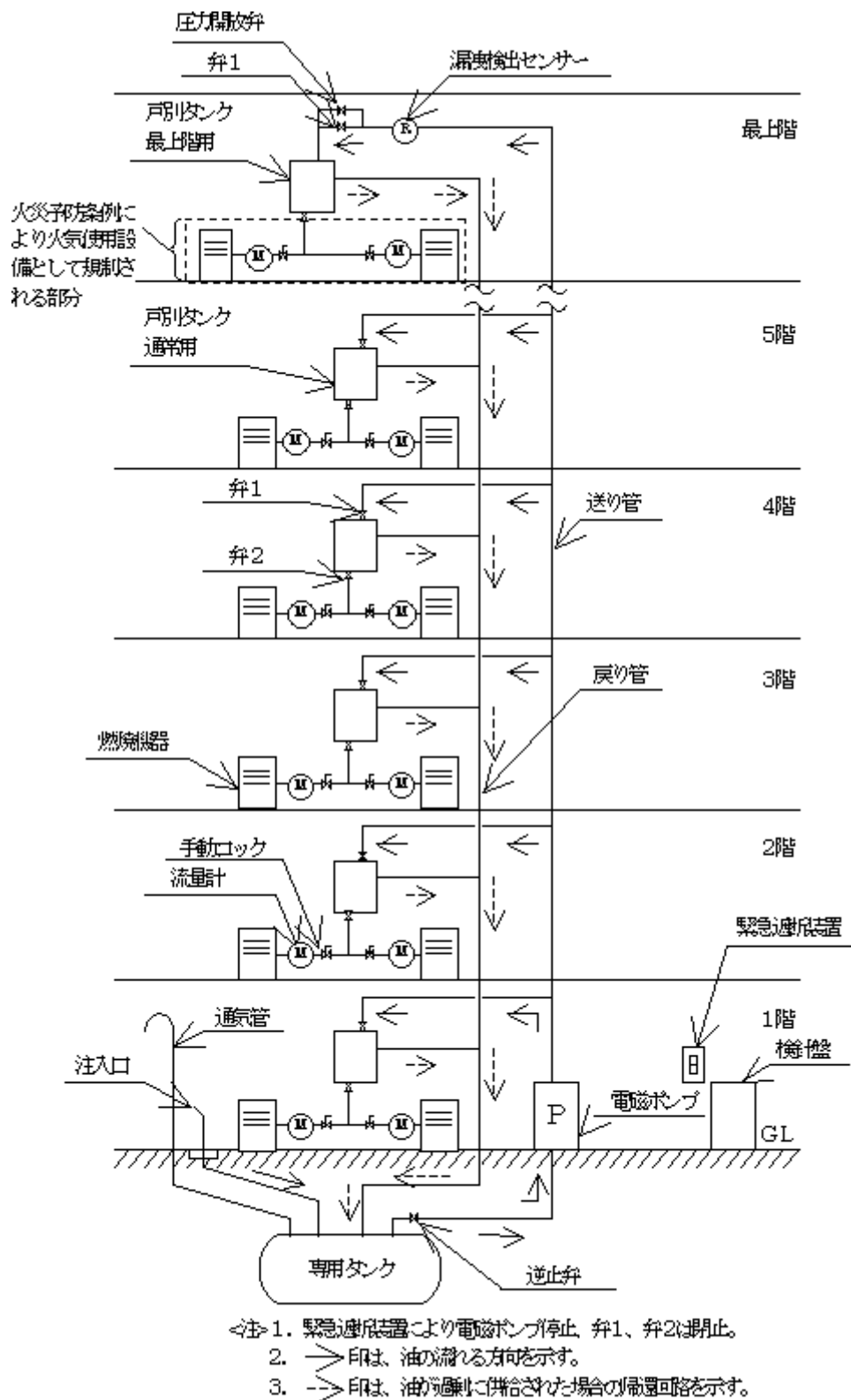
例図5-2 中継タンクを有しない方式の燃料供給施設系統図（系統例2）
