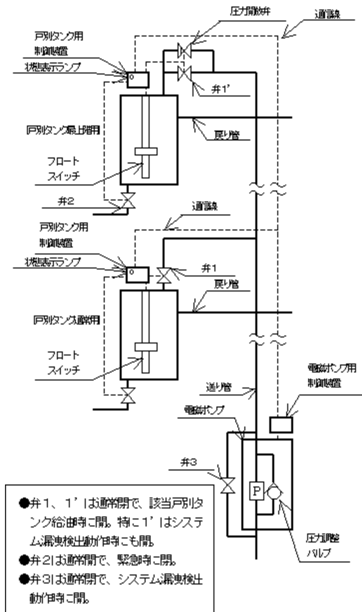
例図 6-2 戸別タンクと電磁ポンプの詳細図（方式例 2）
