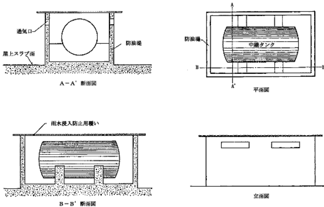
例図3 中継タンクの防油堤概略図
