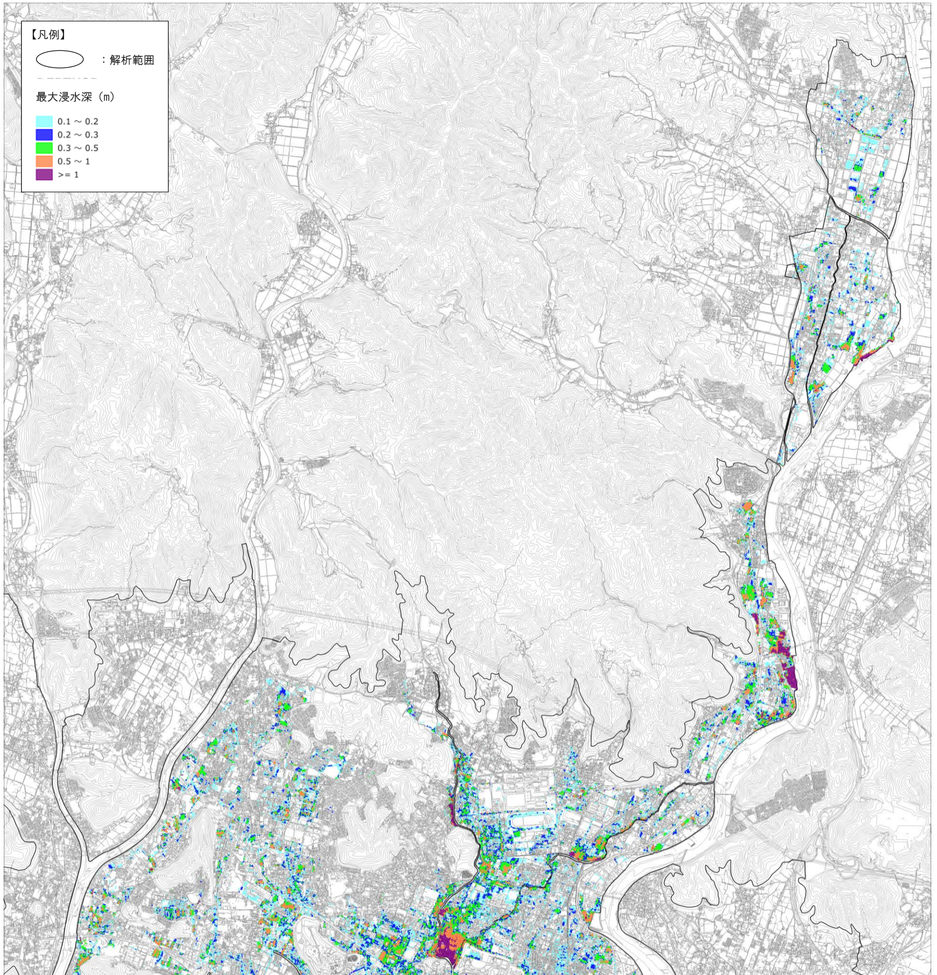
雨水出水浸水想定区域図（中心部北側） 想定最大規模降雨時
