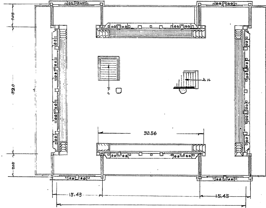
五層平面圖
