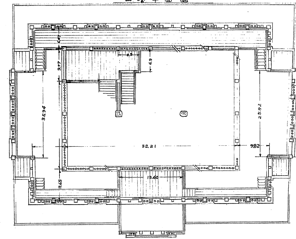
四層平面圖
