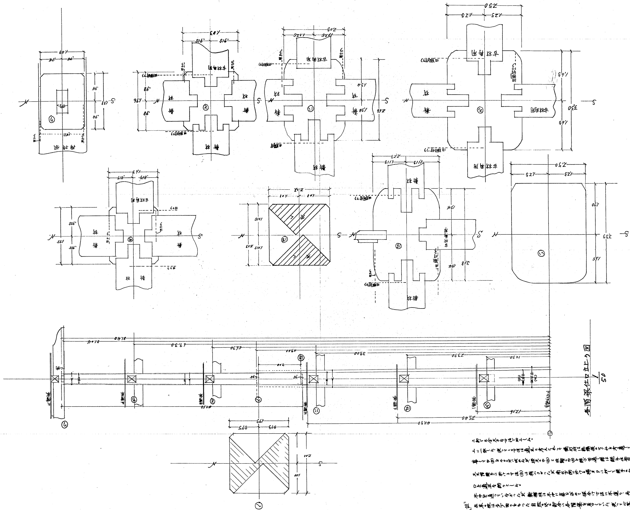
各階床部心材の断面図
