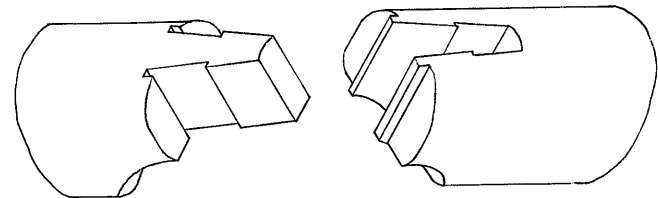
6床梁継手
