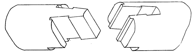
3床梁継手
