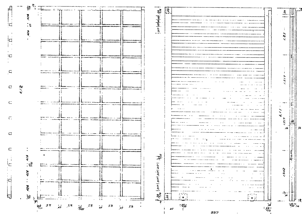
側面平面
