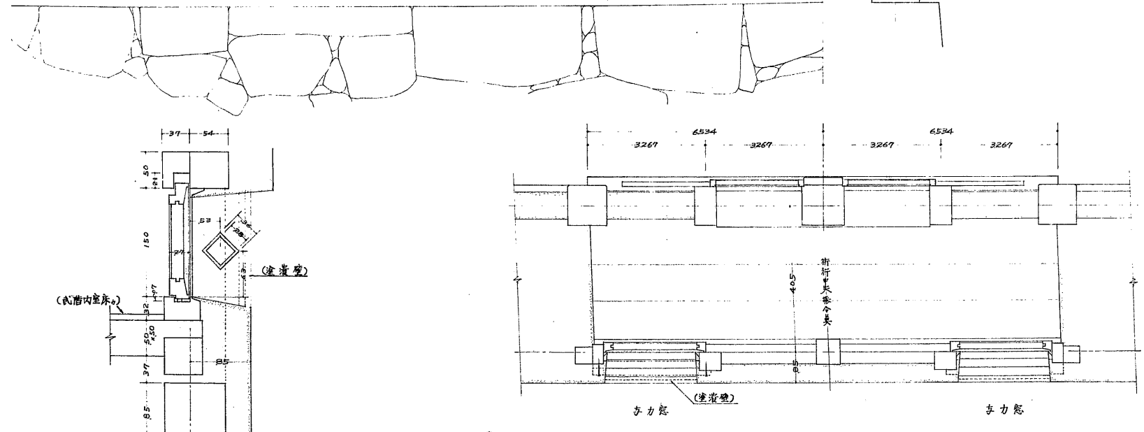
武階東面唐破風内室平面圖 s-6
