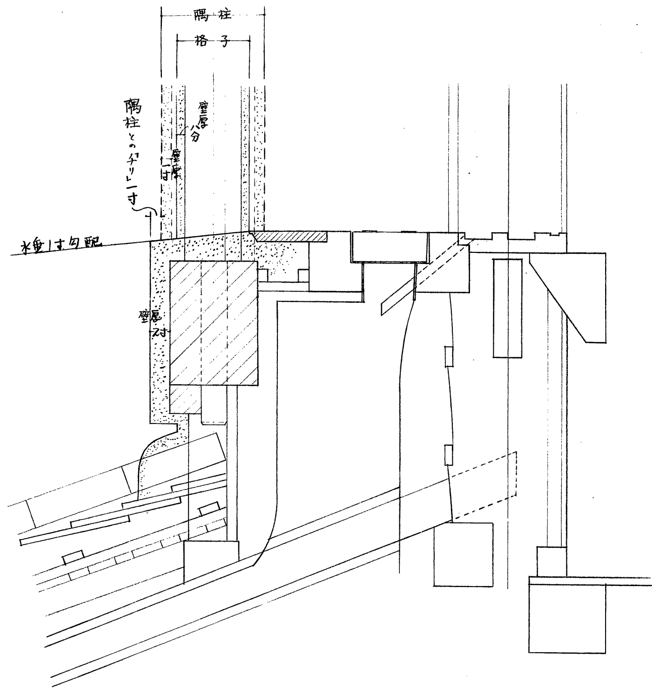
2階南面台格子框壁塗立圖
