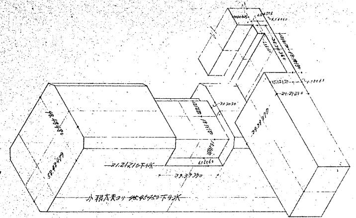
21.8 柱踏梁渡り仕口
