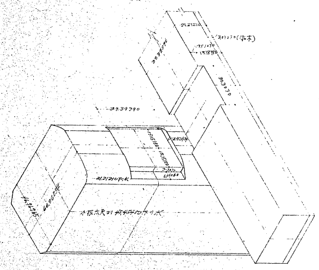
11.3 柱踏梁渡り仕口
