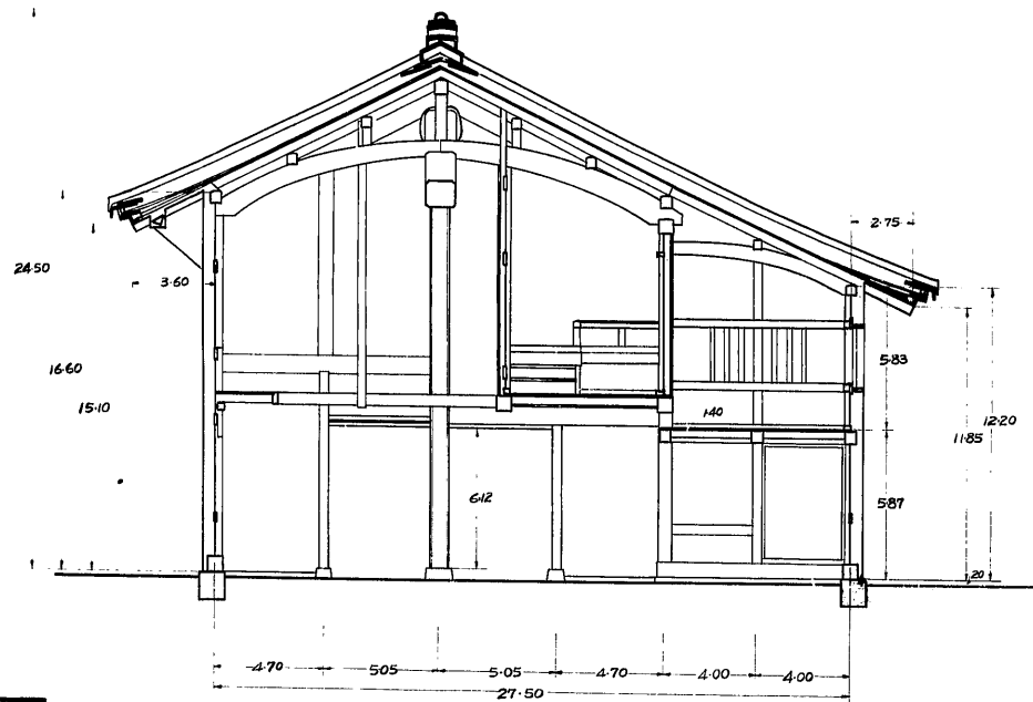
B~B'断面
