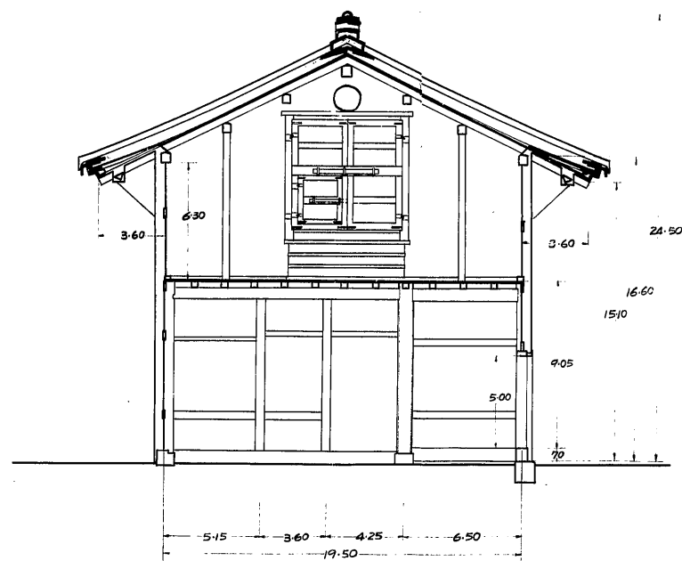
D~D'断面
