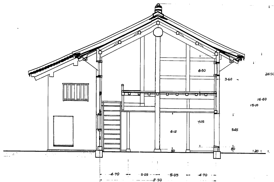
C~C断面
