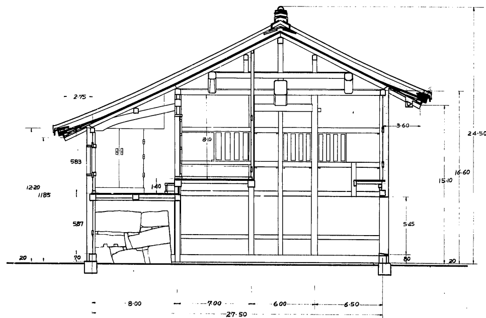
A~A断面
