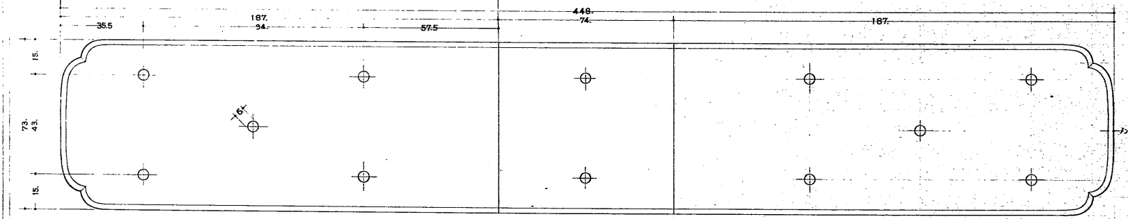
⑯ 飾金物 (階段構) 1ヶ (ハ1)
