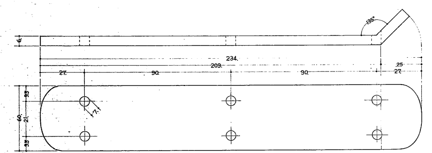
⑰ 飾金物 (階段構) 2ヶ (ハ2)
