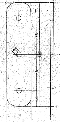
⑦ 飾金物 (階段構) 1ヶ (ハ1)
