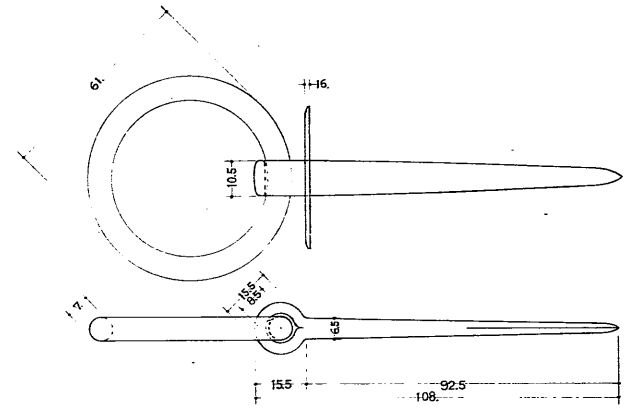
③ 吊 鏢 差金付 (階段構) 3個 (西1・ハ1・ニ1)
