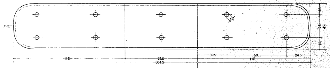
⑥ 飾金物 (階段構) 8ヶ (西4・ハ4)
