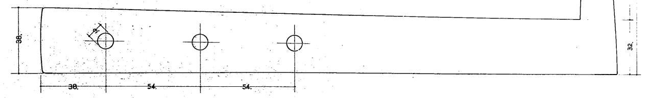
③ 吊 鏢 差金付 (階段構) 3個 (西1・ハ1・ニ1)
