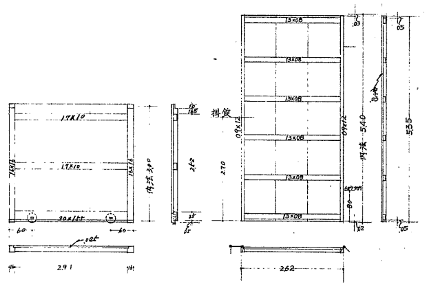
□の渡槽1階南側窓枠 2*(2)
