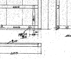
西小天守1階入口風片引扉 1*(4)
