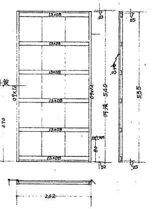
1階の渡槽 風片窓枠 3*(6)
