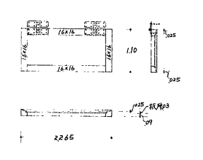
乾小天守2階高窓土戸 2*(1)
