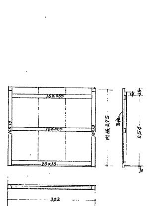
1階の渡槽下屋窓枠(横) 2*(5)
