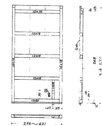
下屋出入口窓枠 7 10.25.28 1*(1) 11.28 1*(2) 12.28 1*(3) 13.28 1*(4) 14.28 1*(5) 15.28 1*(6) 16.28 1*(7)
