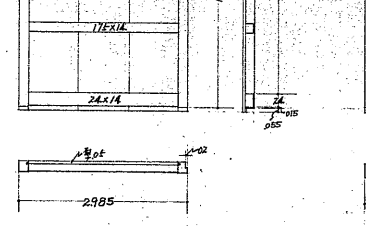
西小天守3階子窓出入口窓枠 1*(3)
