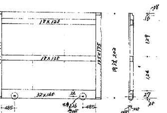
1階の渡槽2階側窓枠 1*(1)
