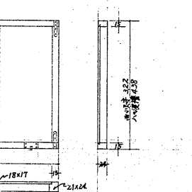
西小天守3階 10.28 1*(2) 11.28 1.0 4.28 2.2 1*(2)
