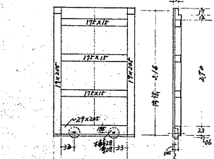
二階橋北側窓枠 2 10.28 1*(3) 11.28 2*(2)
