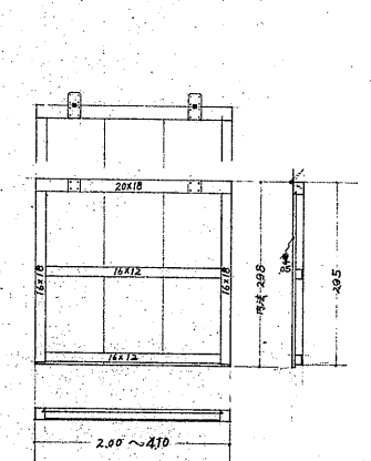
下屋窓枠 10 10.25.28 2*(2) 11.28 2*(1) 12.28 2*(2) 13.28 2*(3) 14.28 2*(4) 15.28 2*(5) 16.28 2*(6) 17.28 2*(7)
