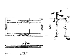
乾小天守4階高窓土戸 1*(2)
