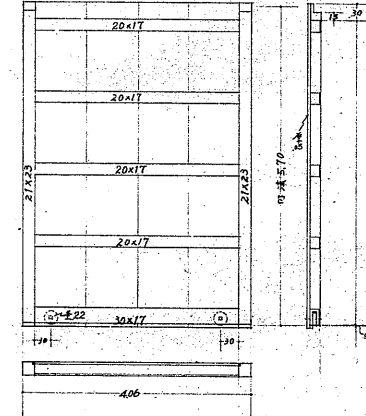
□の渡槽地階入口窓枠 1*(4)
