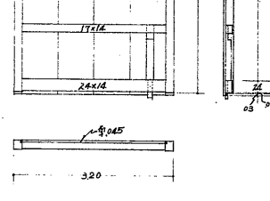
乾小天守3階出入口窓枠 1*(5)
