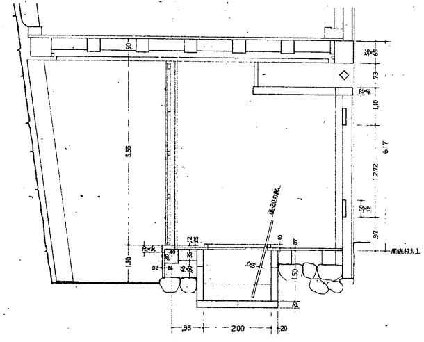
横断面
