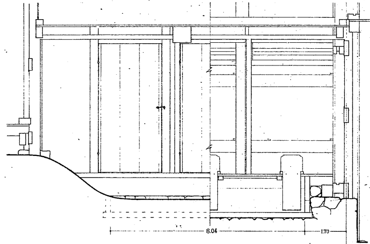
正面・縦断面
