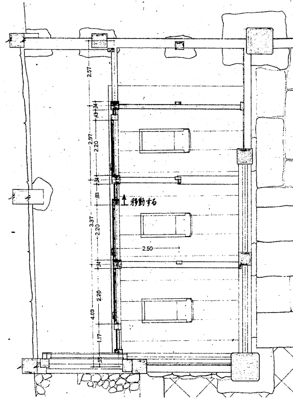
厩現狀 平面
