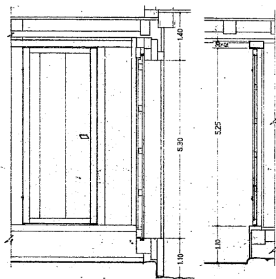
正面 厩現狀 厩出入口
