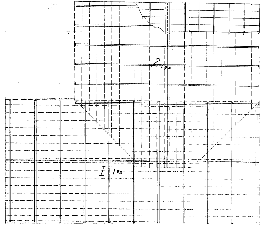
小屋伏図名
