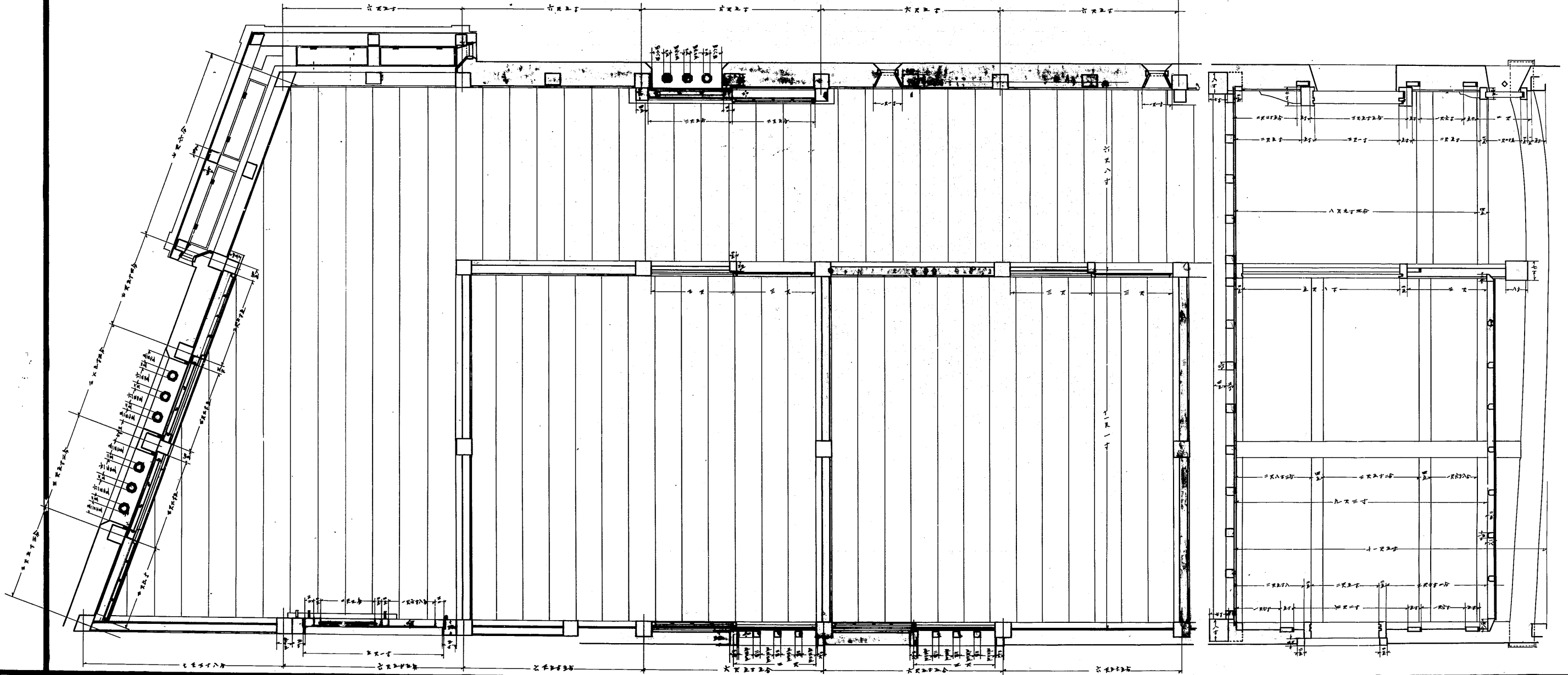
夕、渡槽南部詳細圖 縮尺 貳拾分之二
