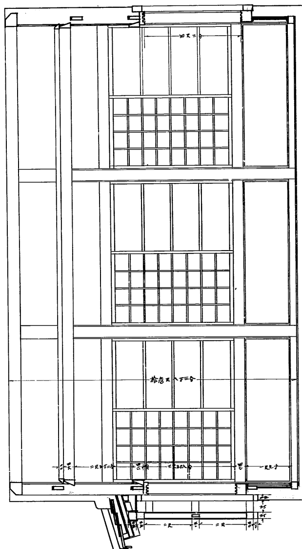
化粧槽現狀變更圖 東面及南面窓詳細圖 縮尺二十分之一
