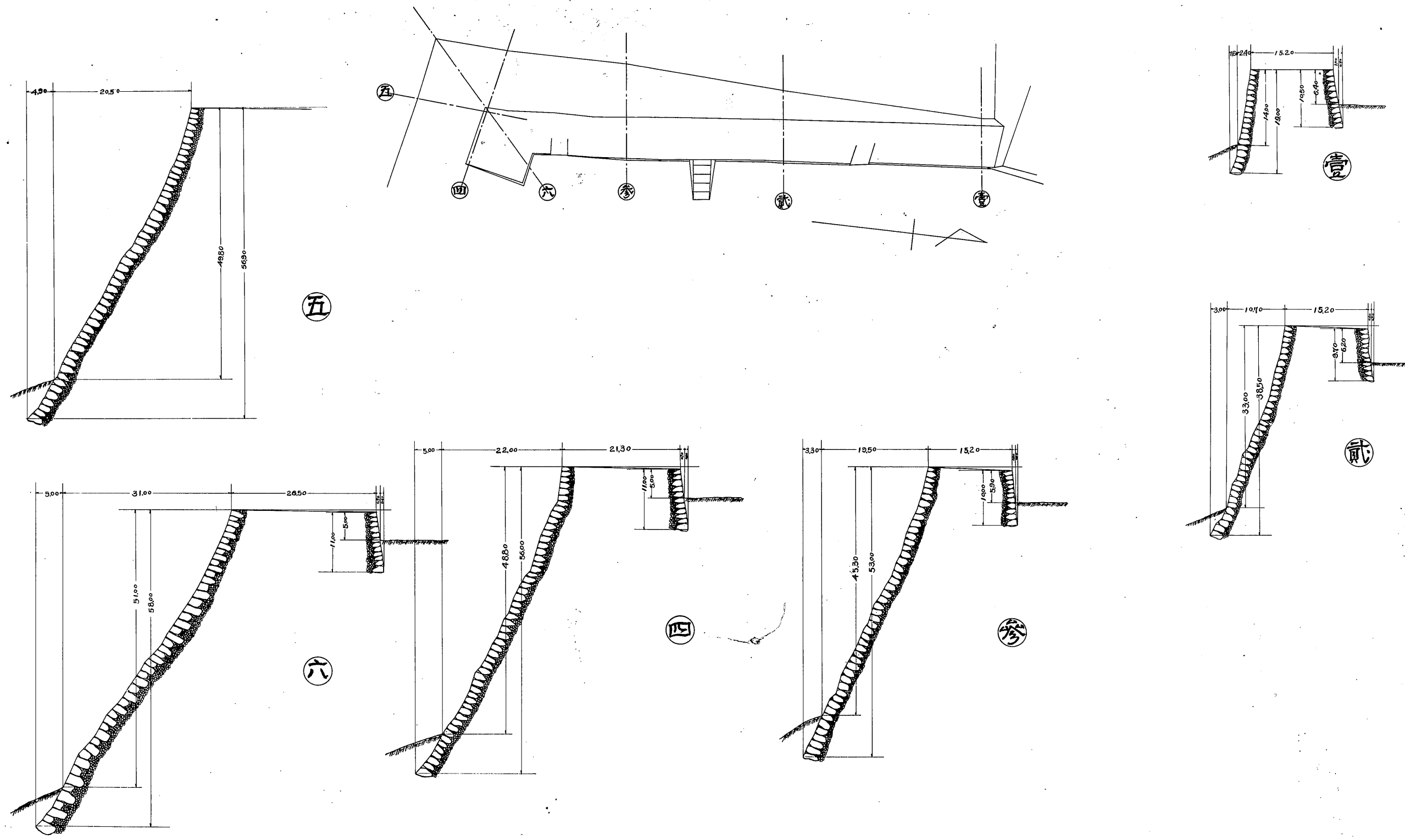
石垣實測断面圖及之槽及L之渡槽 縮尺 百分之壹
