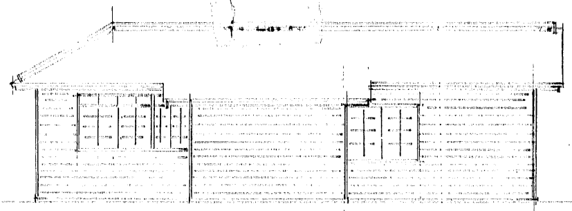
北面立面圖
