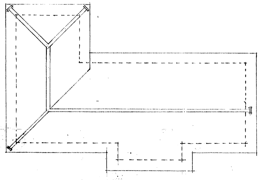
屋根伏圖
