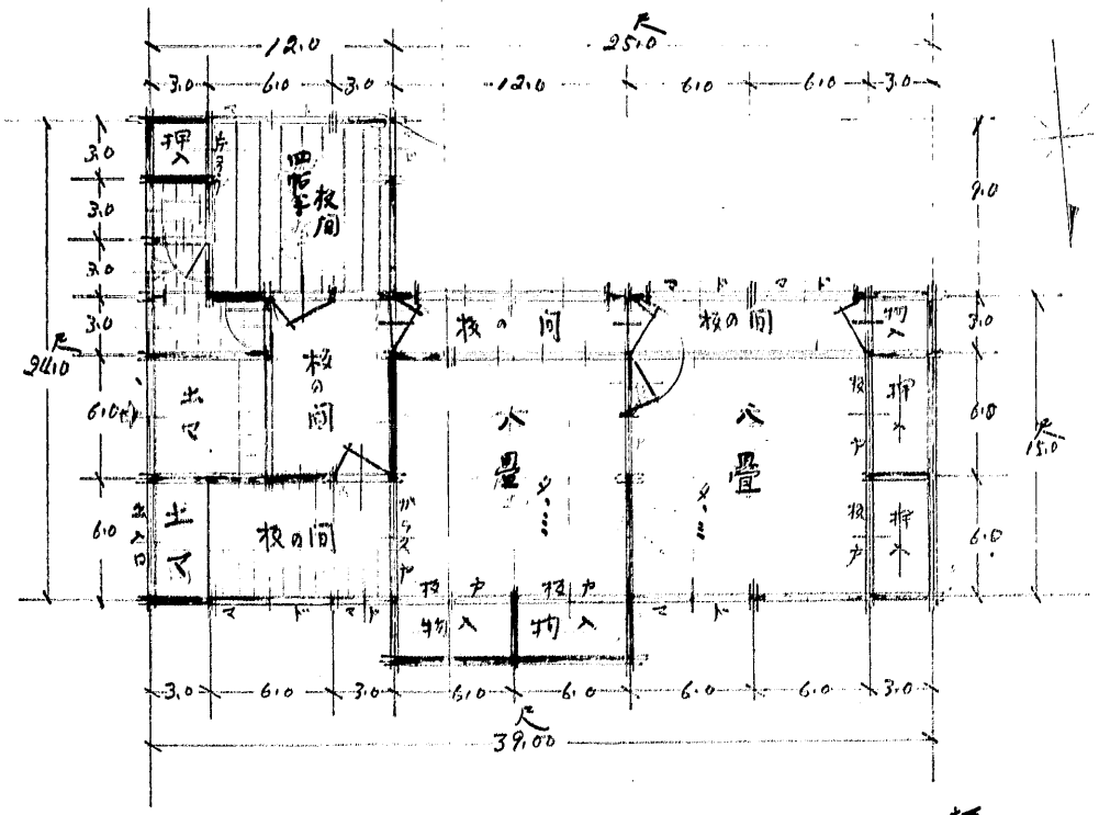
平面圖
