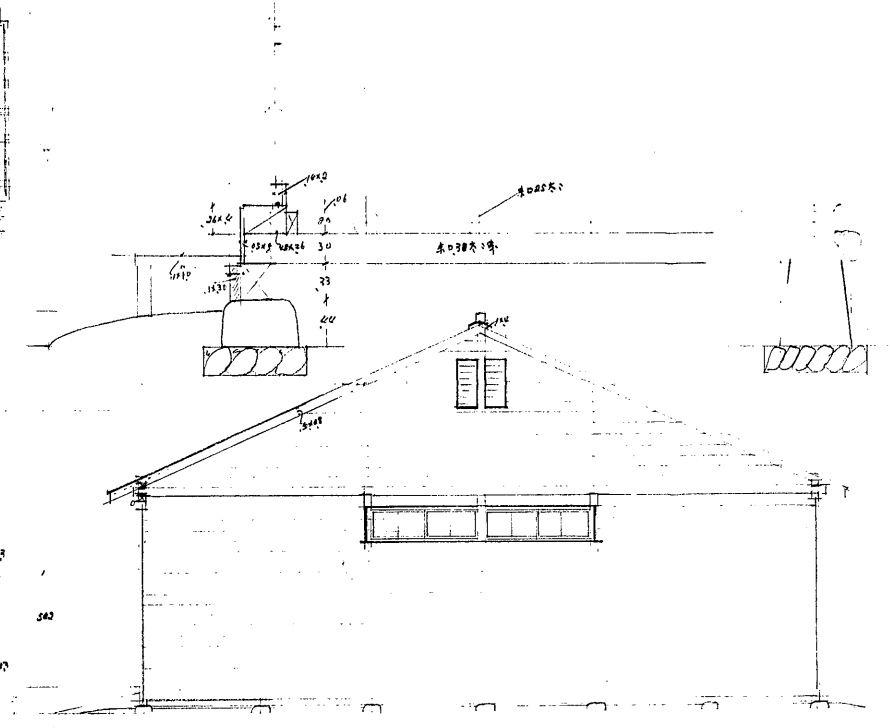
側面等図
