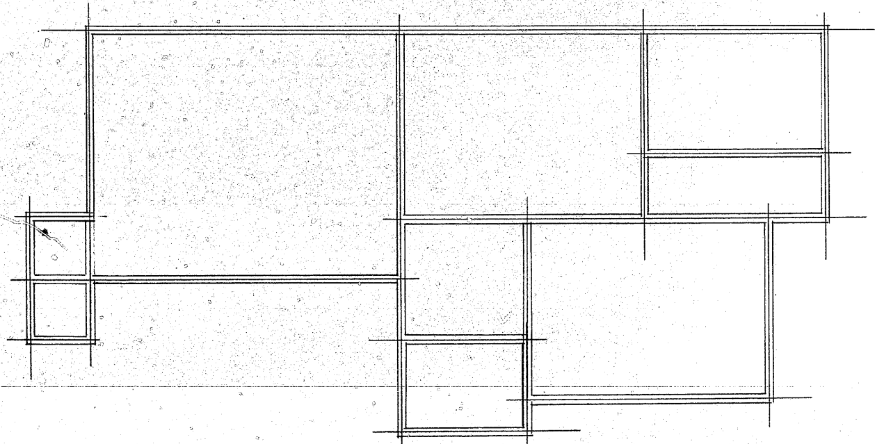
土台伏図
