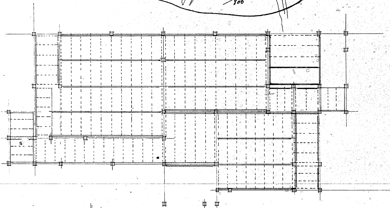
床伏図
