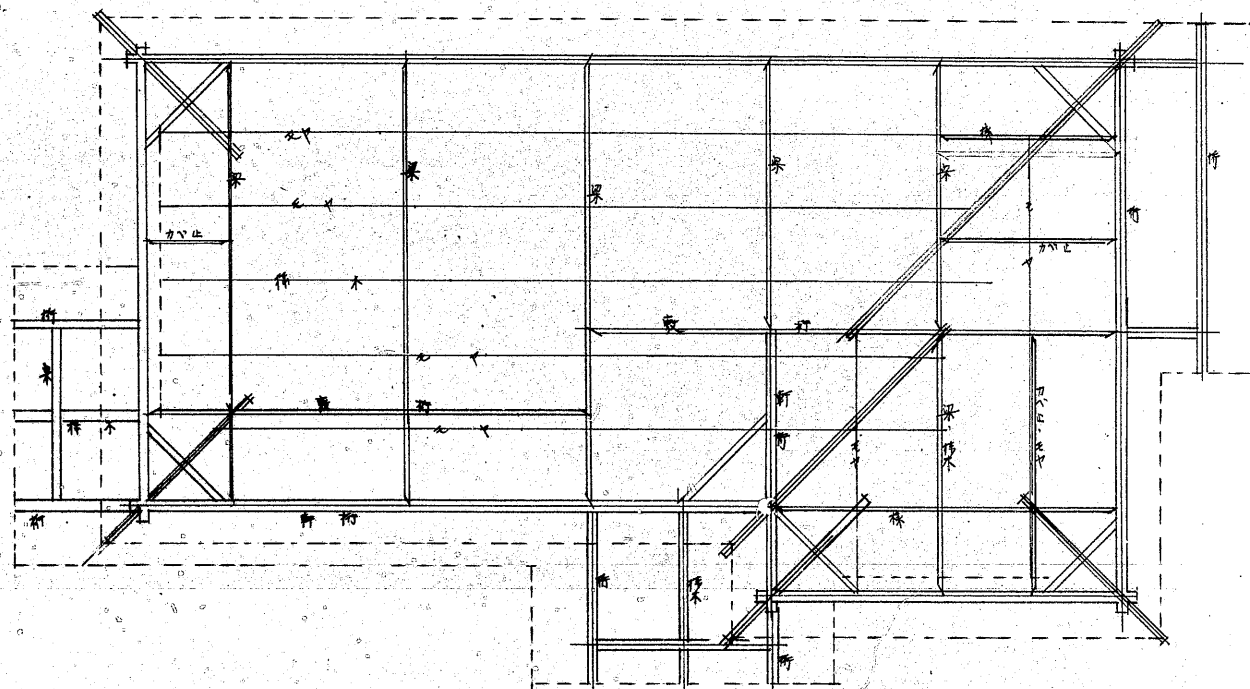
小屋組伏図
