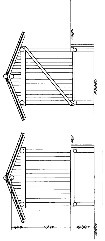
見原番小屋斷面圖
