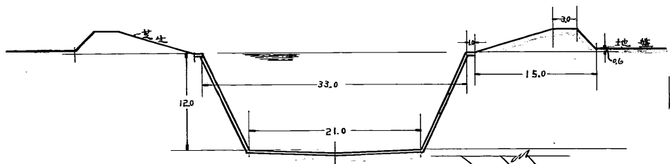
備前及西之丸 断面圖
