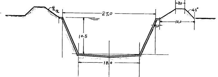
方、櫓東方 断面圖
