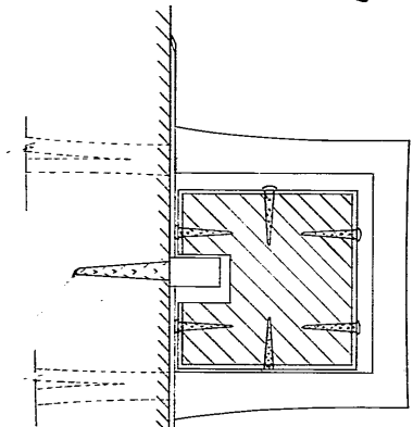
妻戸門金具
