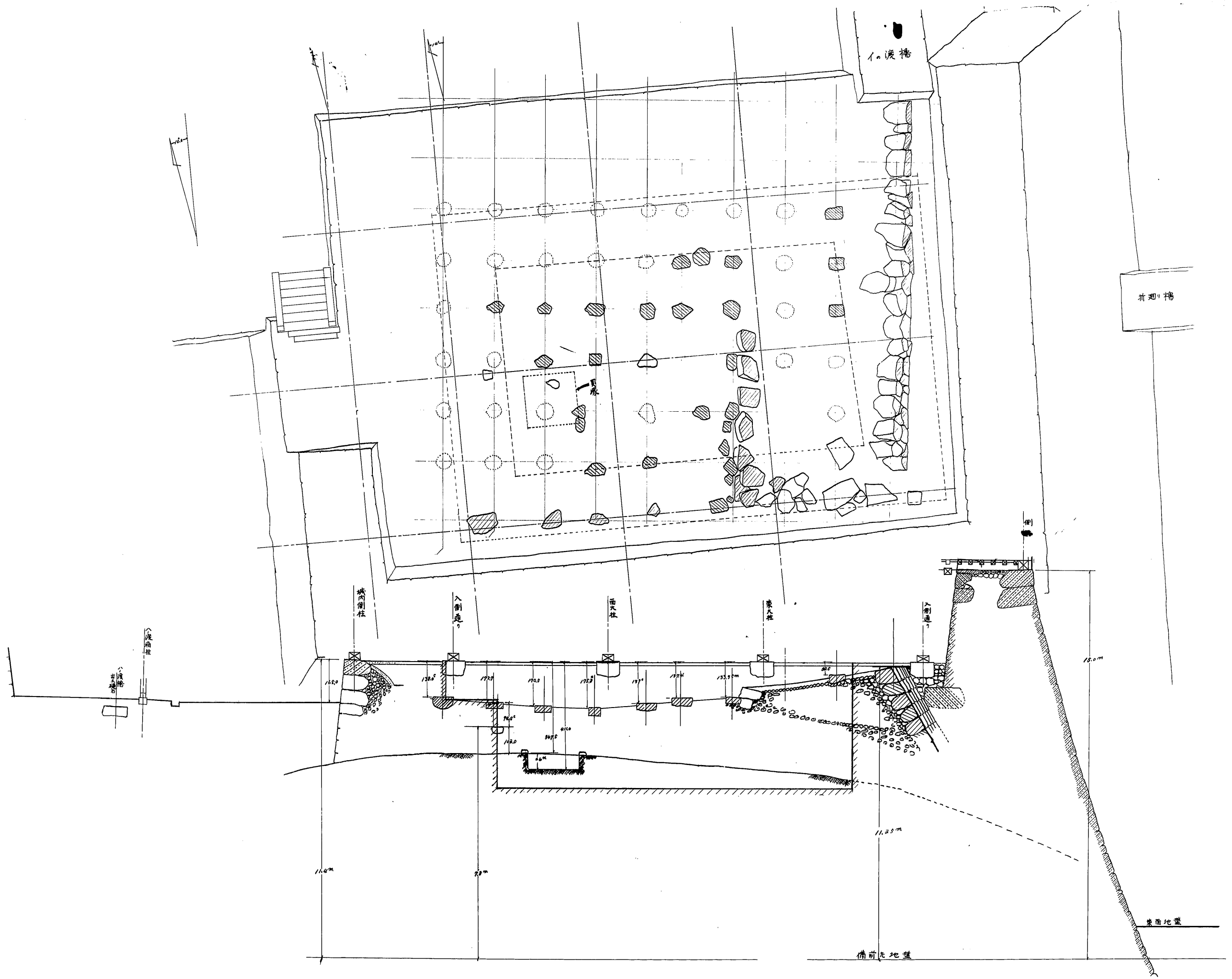
秀吉築造。三重天守出土礎石の配列と東西断面実測図 1/50
