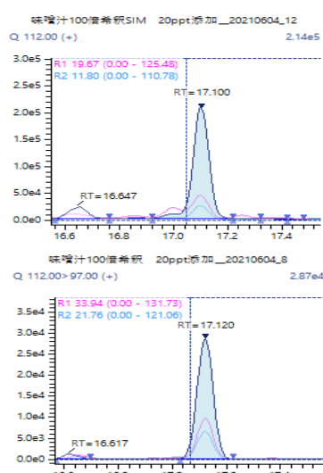
図4 100倍希釈ジェオスミン 比較クロマトグラフ (上が SIM、下が MRM の結果)
