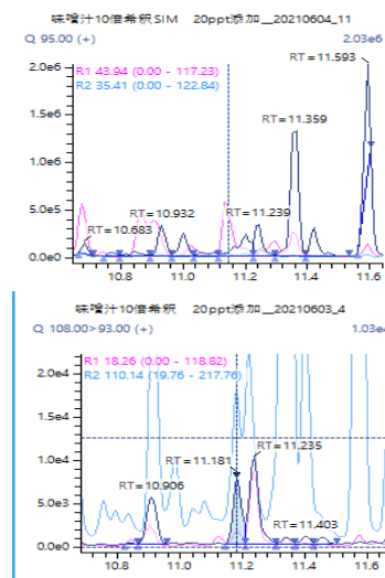
図5 10倍希釈 2-MIB 比較クロマトグラフ (上が SIM、下が MRM の結果)
