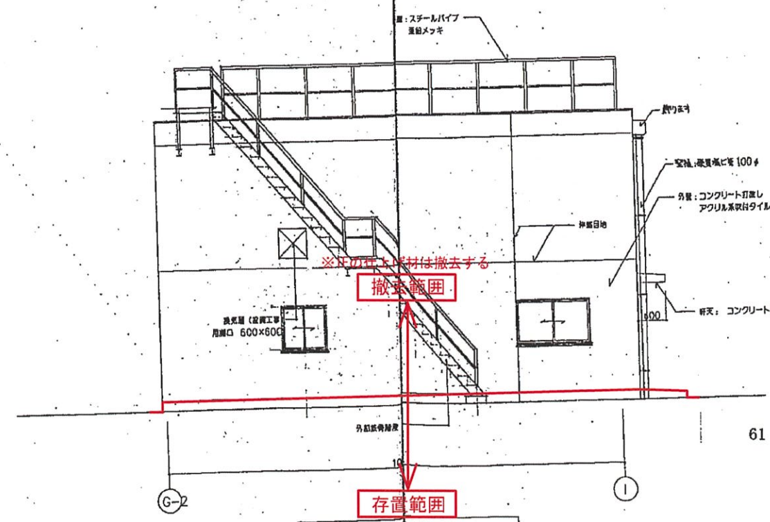
排ガス処理装置室 東立面図 1:50
