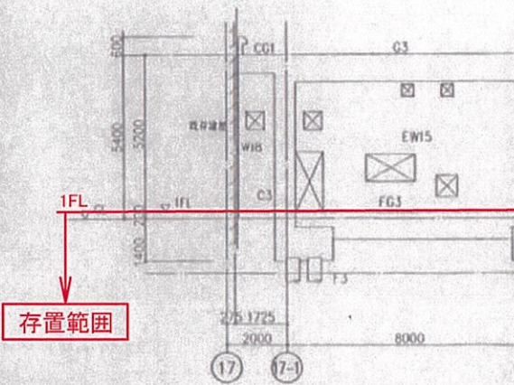
G-2通り輪廻図 1:100
