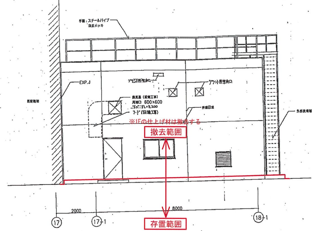
排ガス処理装置室 南立面図 1:50
