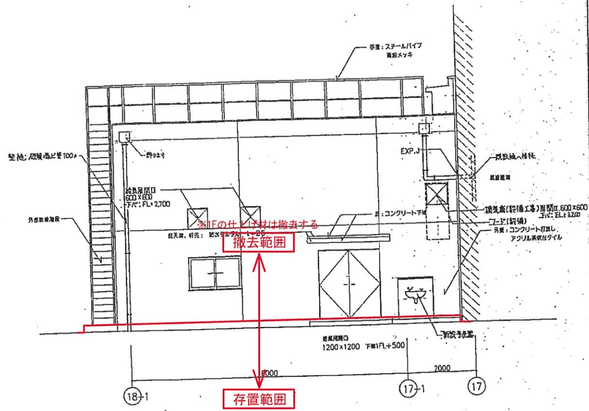
排ガス処理装置室 北立面図 1:50
