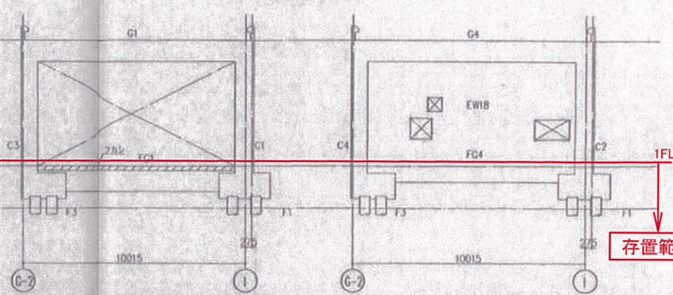
18-1通り輪廻図 1:100
