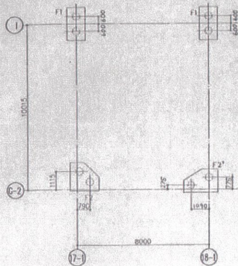
机·基礎伏圖 1:100
