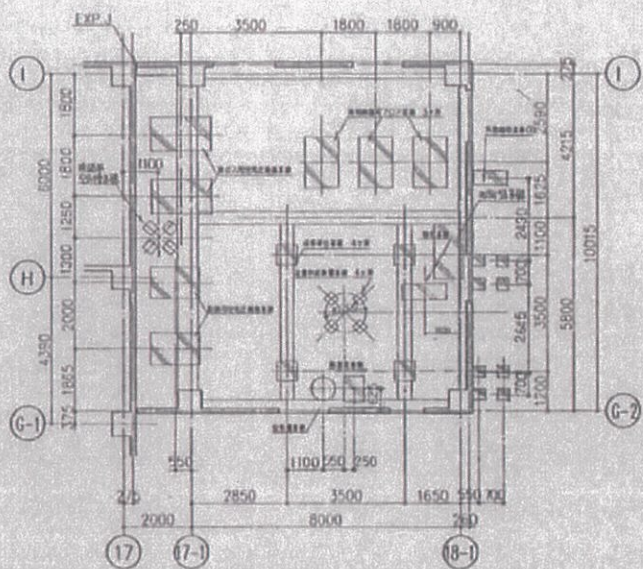
机械基础位置图 1:100
