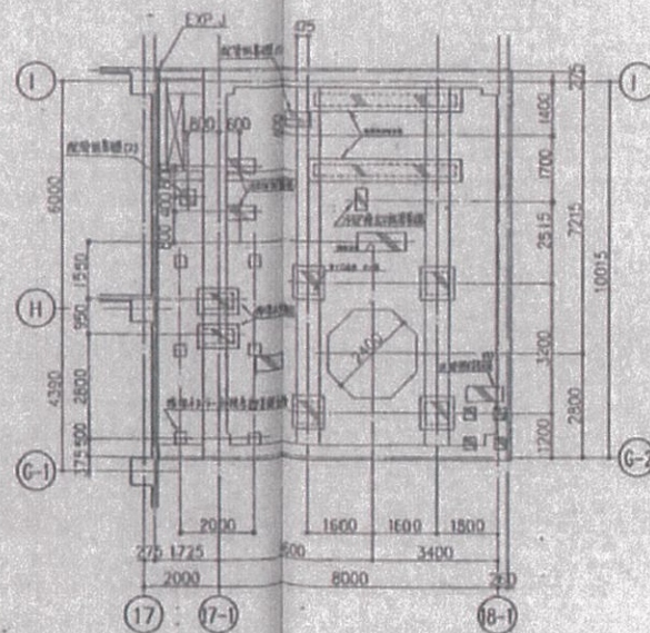
地基基礎位置圖 1:100
