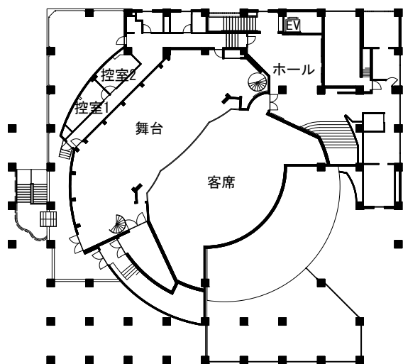
5 階平面図
