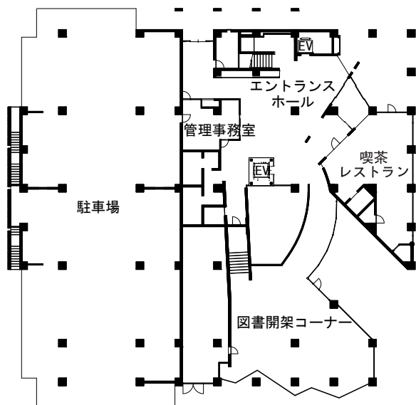
1 階平面図
