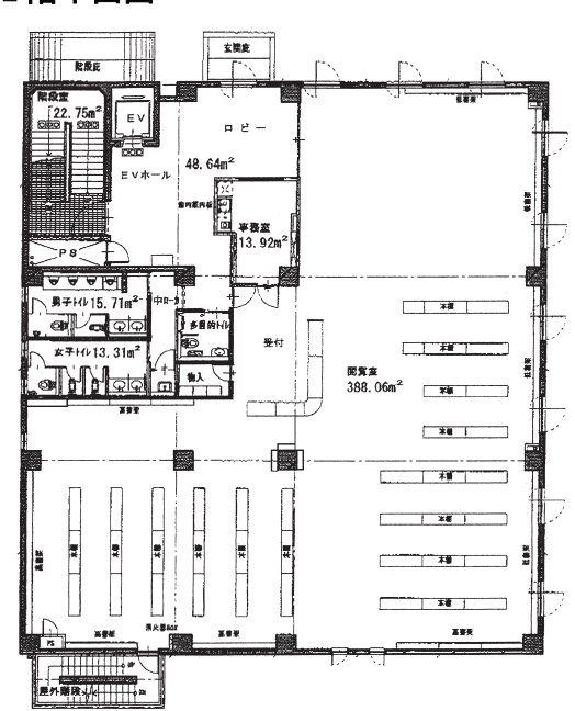
2階平面図
