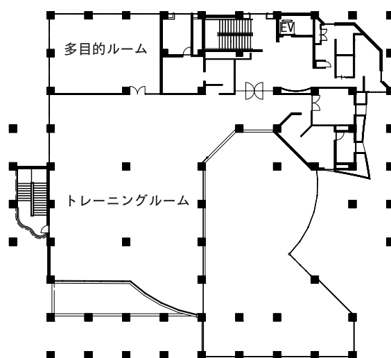
4 階平面図
