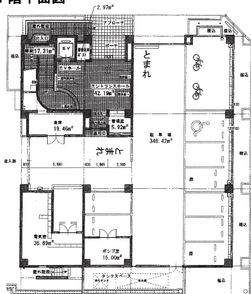
1 階平面図
