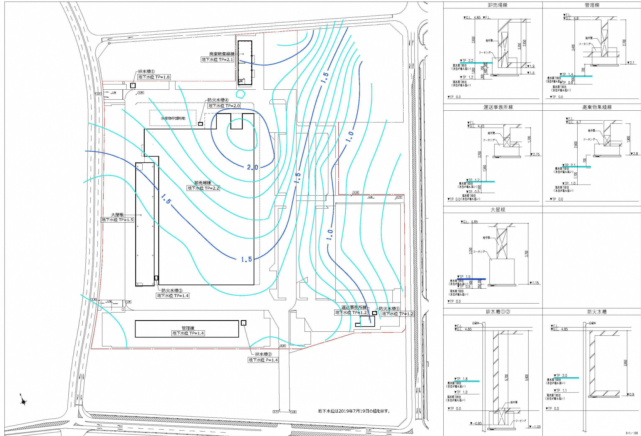
建屋と地下水位の関係
