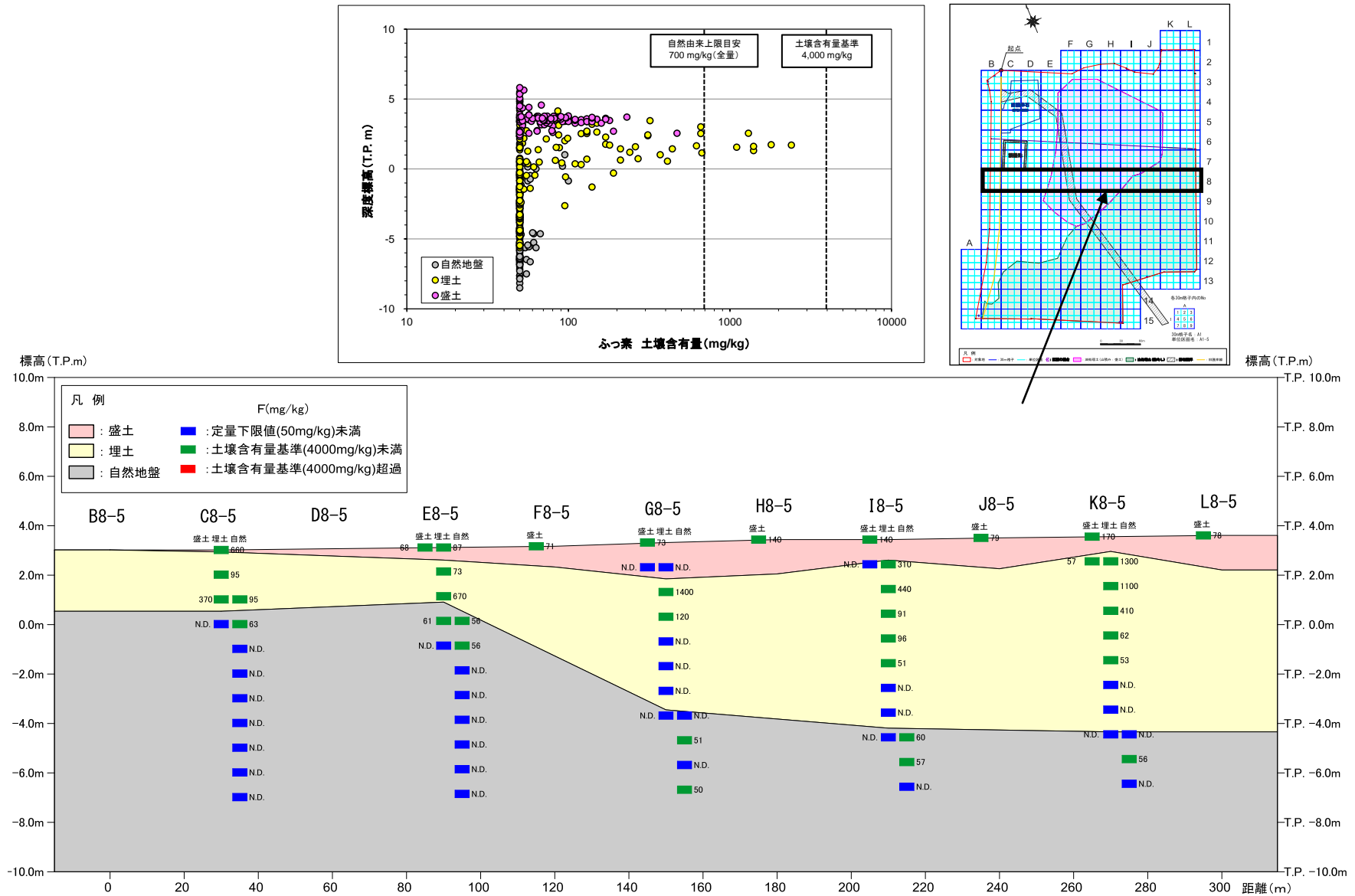
図 8. 1. 23 ふっ素土壌含有量の深度別基準超過状況 (代表 : 8 の 30m 格子行)
