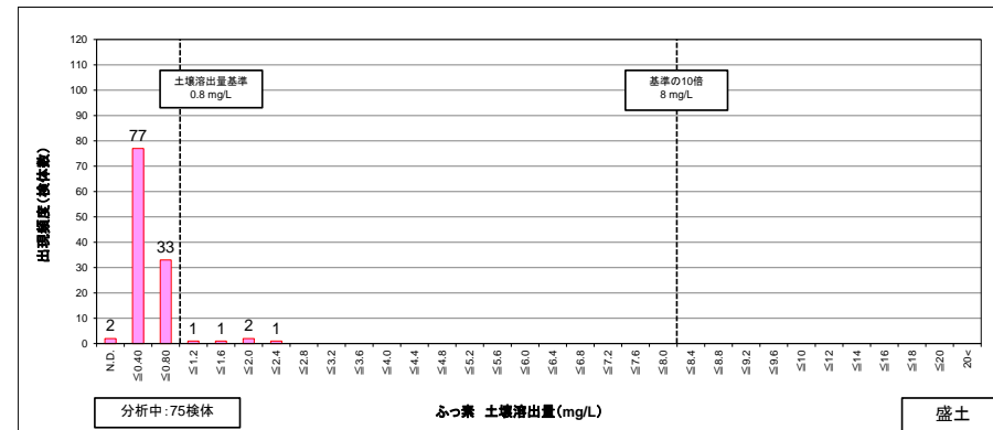
図 8.1.18 (1) 盛土におけるふっ素土壌溶出量の検出頻度分布
