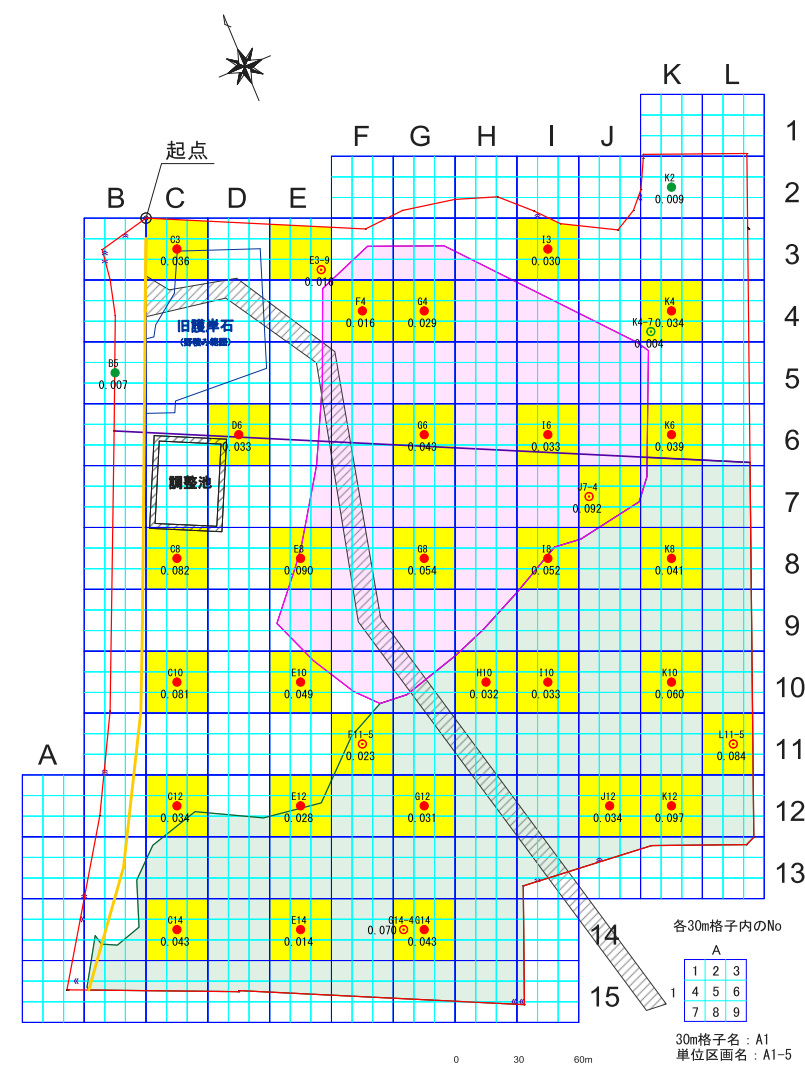
図 8.1.13 (2) 埋土における砒素土壤溶出量の検出頻度分布
