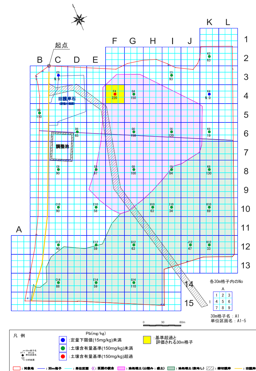
図 8.1.7 (3) 自然地盤における鉛土壌含有量の平面分布
