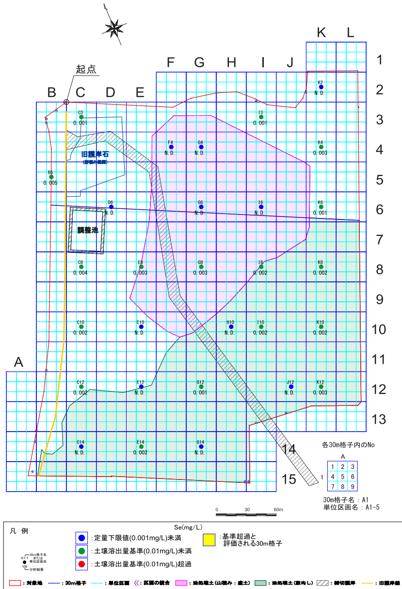
図 8.1.31 (1) 埋土におけるセレン土壌溶出量の平面分布
