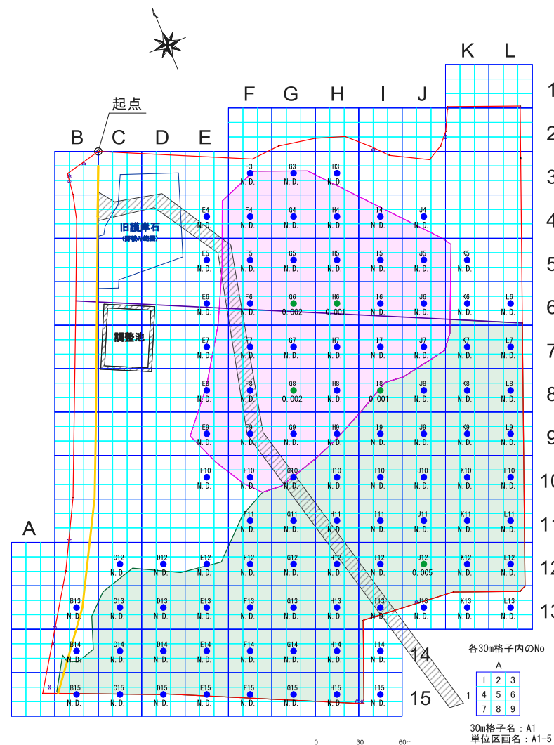
図 8.1.4 (1) 盛土における鉛土壌溶出量の検出頻度分布
