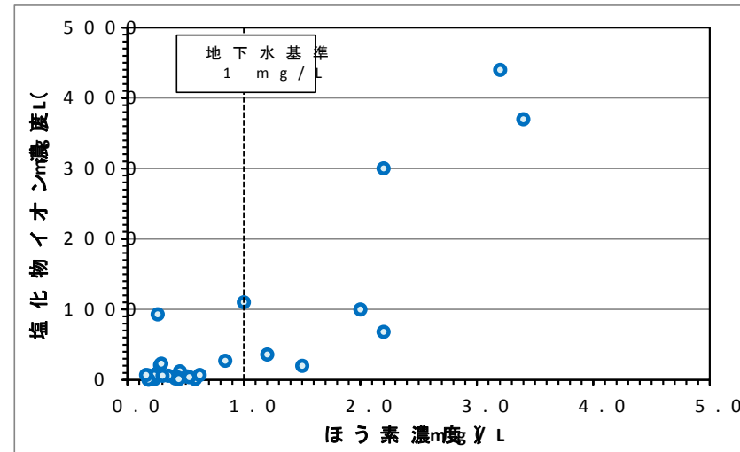
図 8.2.5 塩化物イオンと硝素、ふっ素、ほう素地下水濃度の関係
