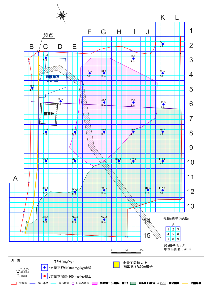
図 8.1.38 (3) 自然地盤における TPH (C6-C44) の平面分布
