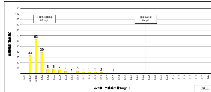
図 8.1.18 (2) 埋土におけるふっ素土壌溶出量の検出頻度分布
