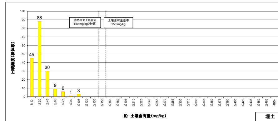
図 8.1.6 (2) 埋土における鉛土壌含有量の検出頻度分布
