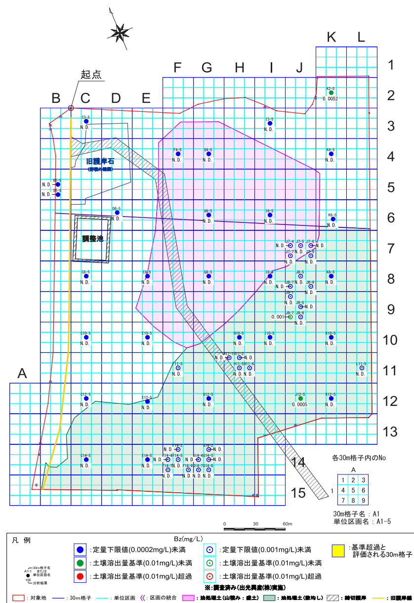
図 8.1.2 (4) 自然地盤におけるベンゼン土壌溶出量の平面分布
