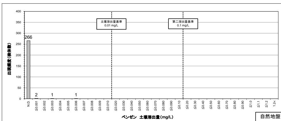
図 8.1.1 (3) 自然地盤におけるベンゼン土壌溶出量の検出頻度分布
