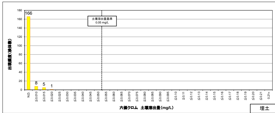
図 8.1.27 (1) 埋土における六価クロム土壌溶出量の検出頻度分布
