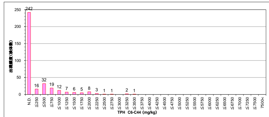
図 8.1.37 (1) 盛土における TPH (C6-C44) の検出頻度分布
