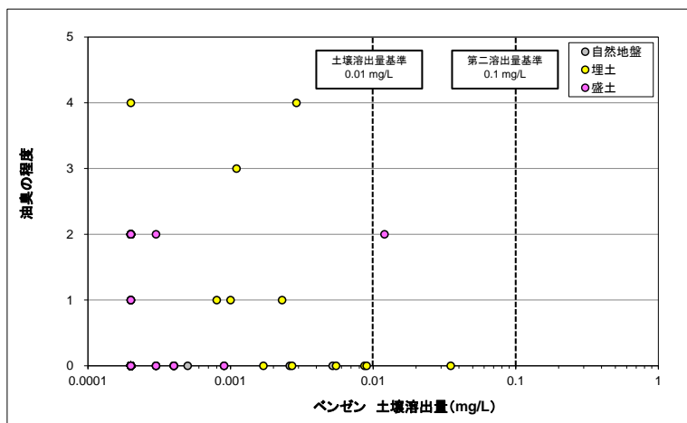
図 8. 1. 41 (2) ベンゼン土壌溶出量と油分の関係 (油臭の程度)
