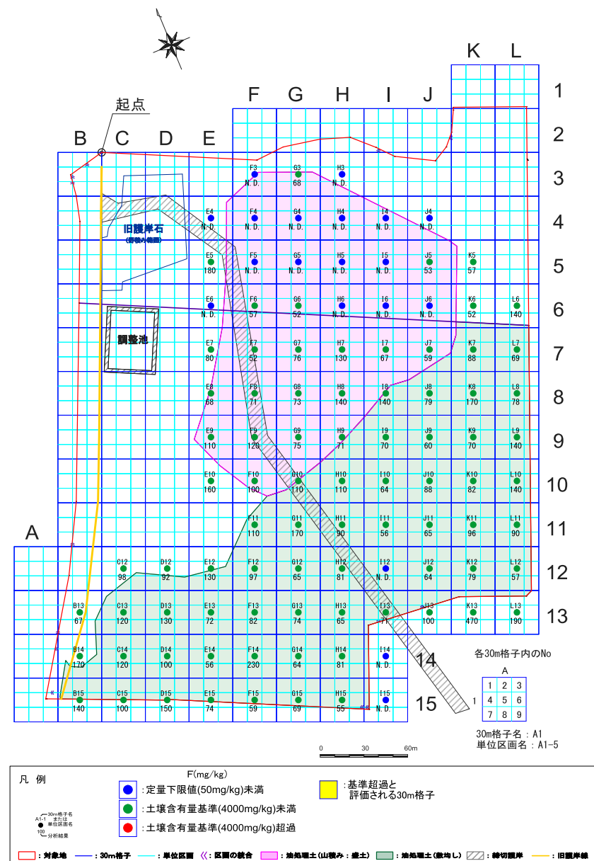
図 8.1.21 (1) 盛土におけるふっ素土壌含有量の平面分布
