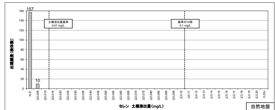
図 8.1.28 (2) 自然地盤におけるセレン土壌溶出量の検出頻度分布
