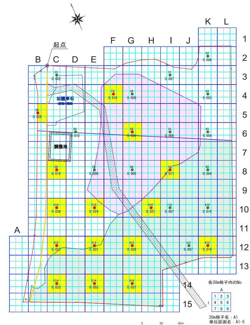
図 8.1.4 (3) 自然地盤における鉛土壌溶出量の検出頻度分布
