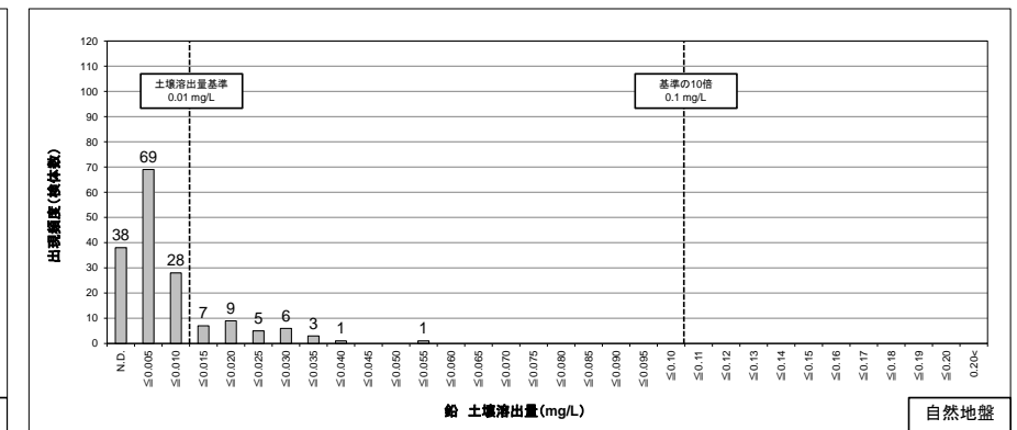
図 8.1.4 (3) 自然地盤における鉛土壌溶出量の検出頻度分布
