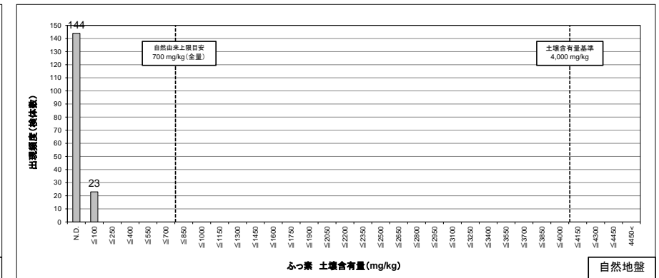
図 8.1.20 (3) 自然地盤におけるふっ素土壌含有量の検出頻度分布
