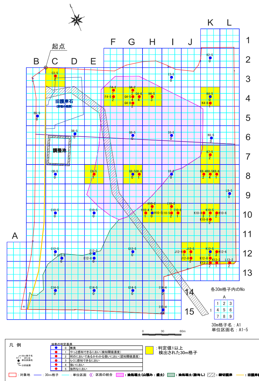
図 8.1.34 (2) 埋土における油臭の程度の平面分布
