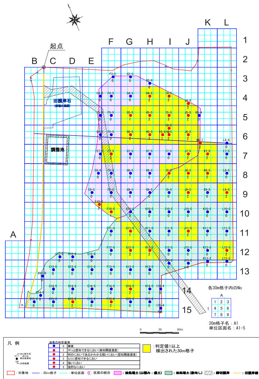
図 8.1.34 (1) 盛土における油臭の程度の平面分布
