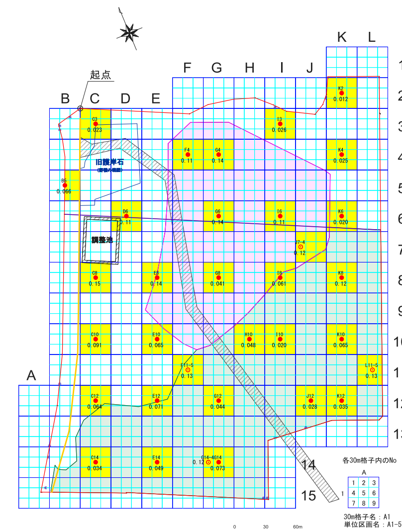
図 8.1.13 (3) 自然地盤における砒素土壤溶出量の検出頻度分布
