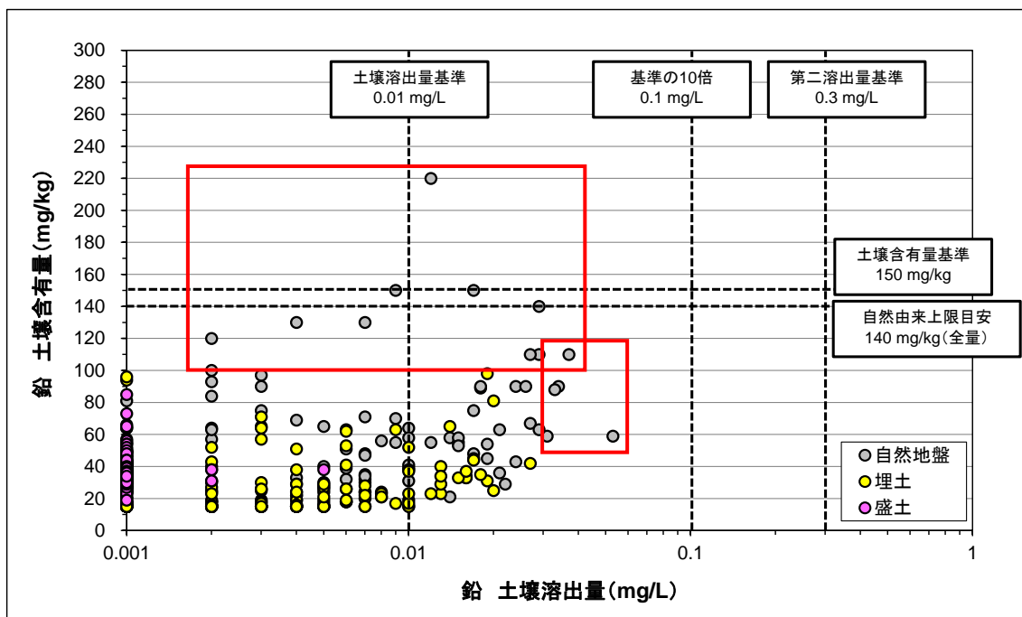
図 8.1.12 鉛土壤溶出量と鉛土壤含有量の関係
