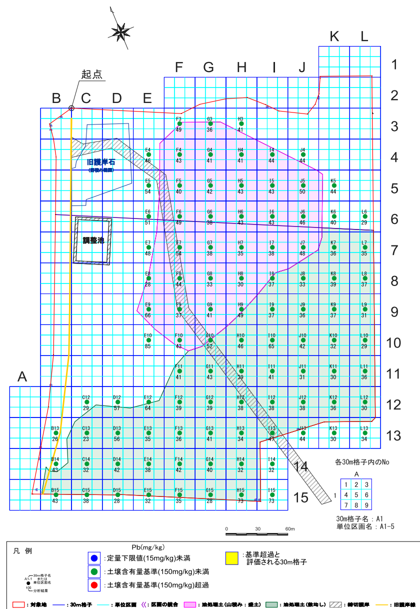
図 8.1.7 (1) 盛土における鉛土壌含有量の平面分布
