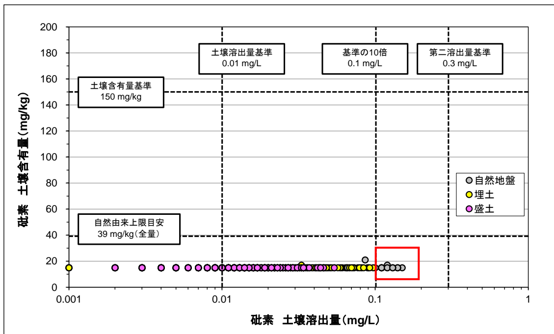
図 8.1.17 砒素土壌溶出量と砒素土壌含有量の関係
