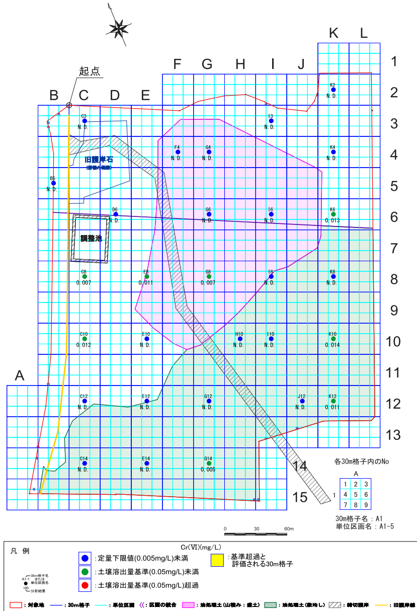
図 8.1.30 (1) 埋土における六価クロム土壤溶出量の平面分布
