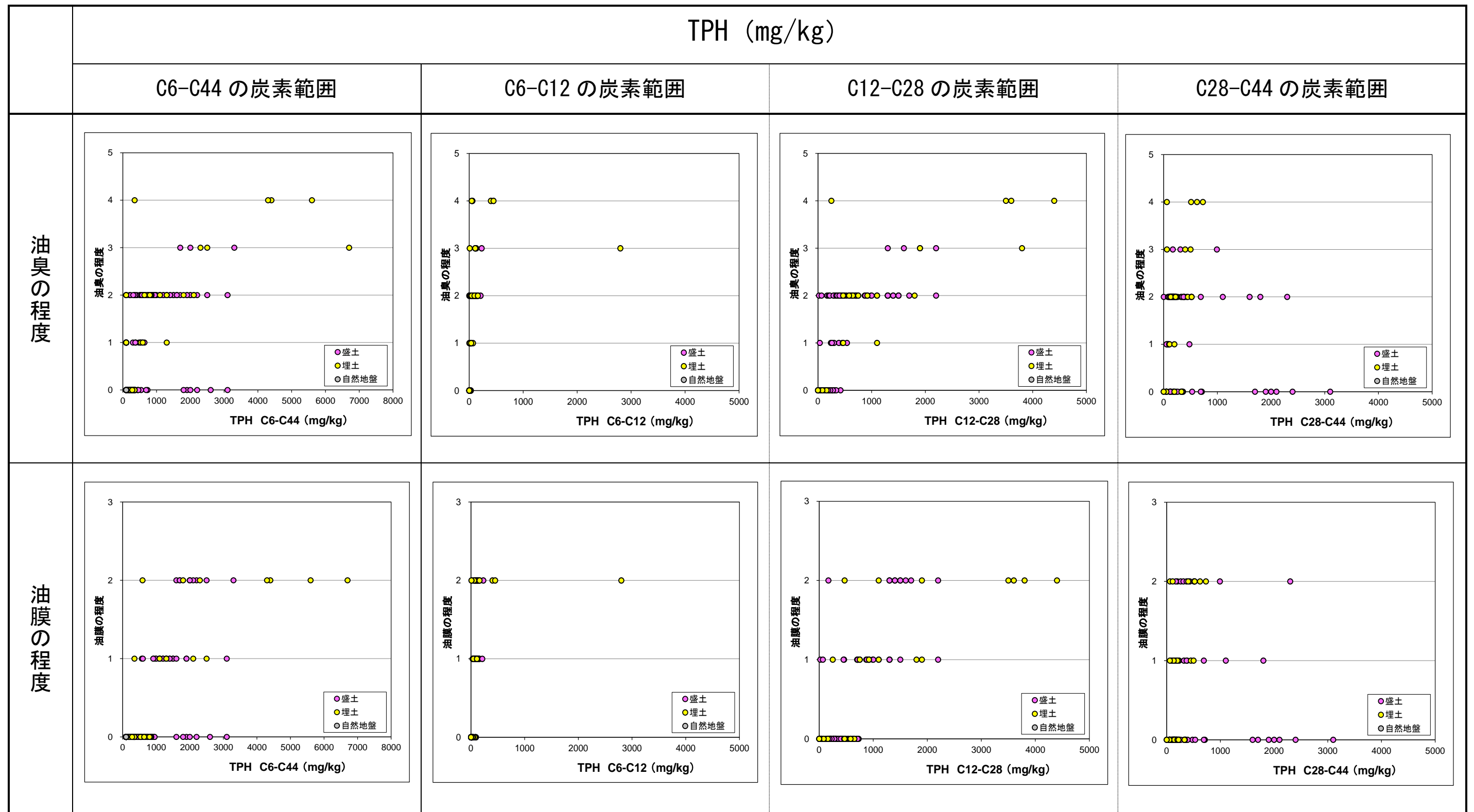
図 8.1.40 TPH と油臭・油膜の関係
