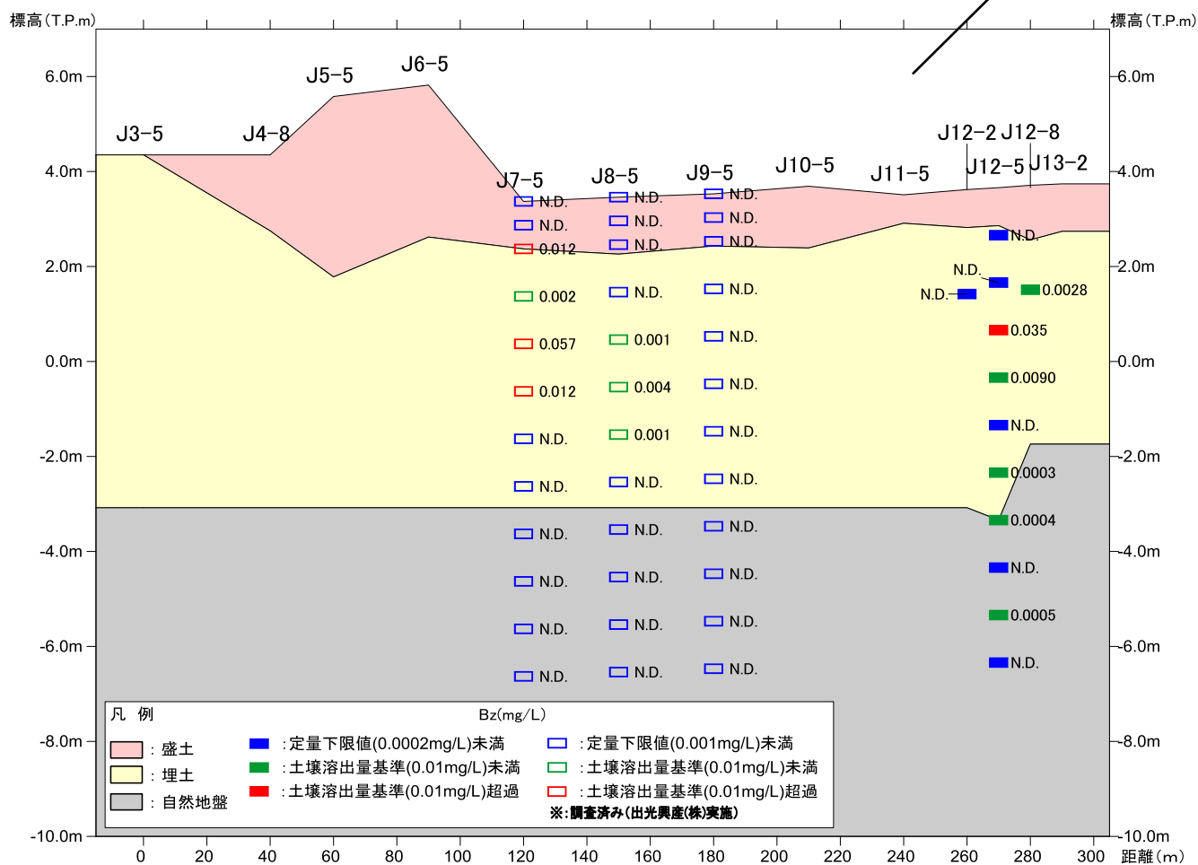
図 8.1.3 ベンゼン土壌溶出量の深度別基準超過状況 (代表: J の 30m 格子列)
