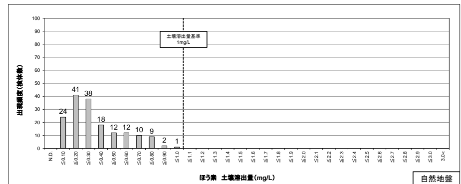
図 8.1.29 (2) 自然地盤におけるほう素土壌溶出量の検出頻度分布
