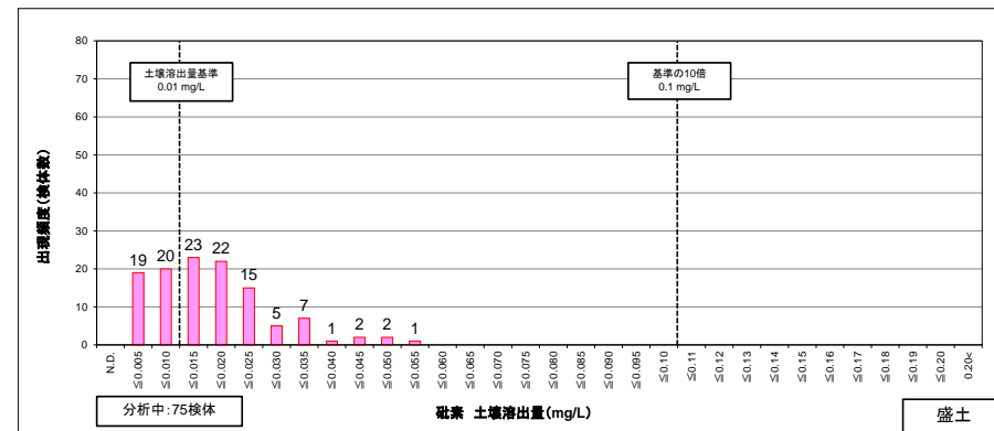
図 8.1.13 (1) 盛土における砒素土壤溶出量の検出頻度分布
