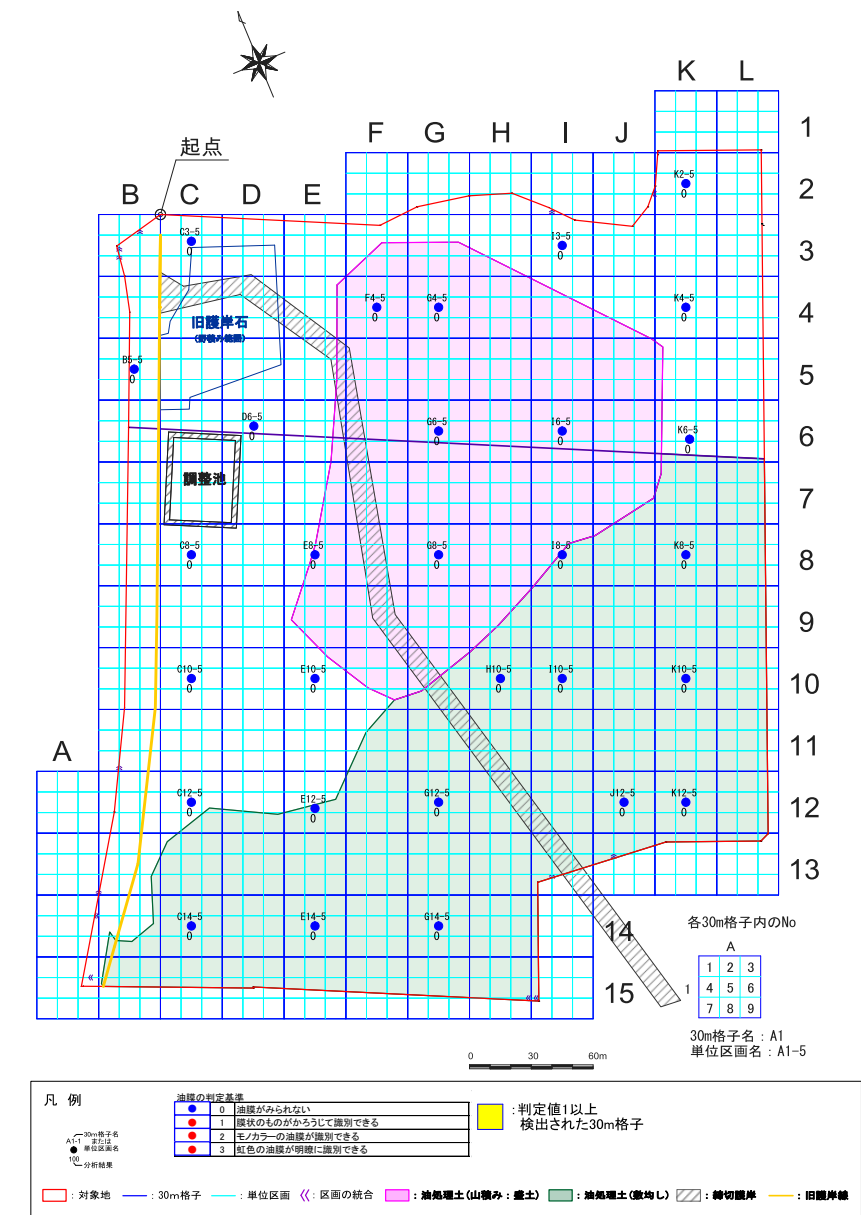
図 8.1.36 (3) 自然地盤における油膜の程度の平面分布
