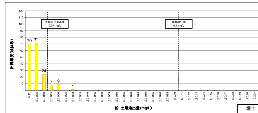
図 8.1.4 (2) 埋土における鉛土壌溶出量の検出頻度分布
