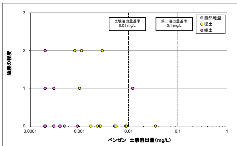
図 8. 1. 41 (2) ベンゼン土壌溶出量と油分の関係 (油膜の程度)
