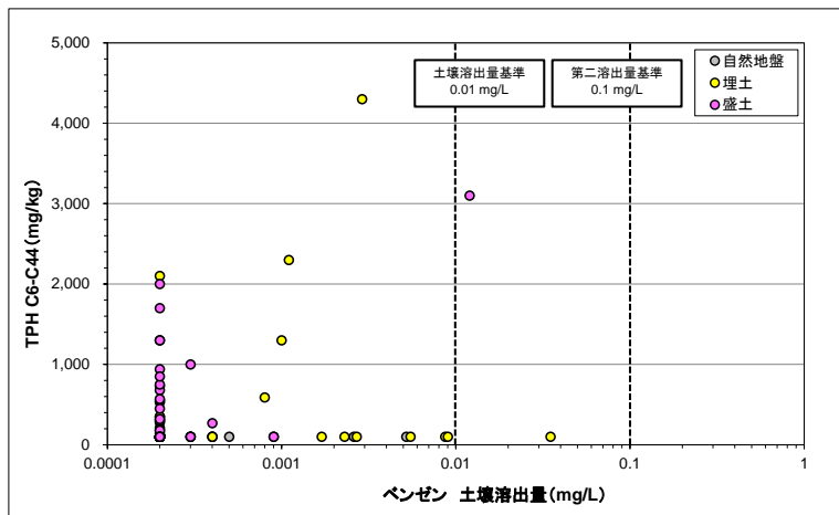
図 8. 1. 41 (1) ベンゼン土壌溶出量と油分の関係 (TPH)
