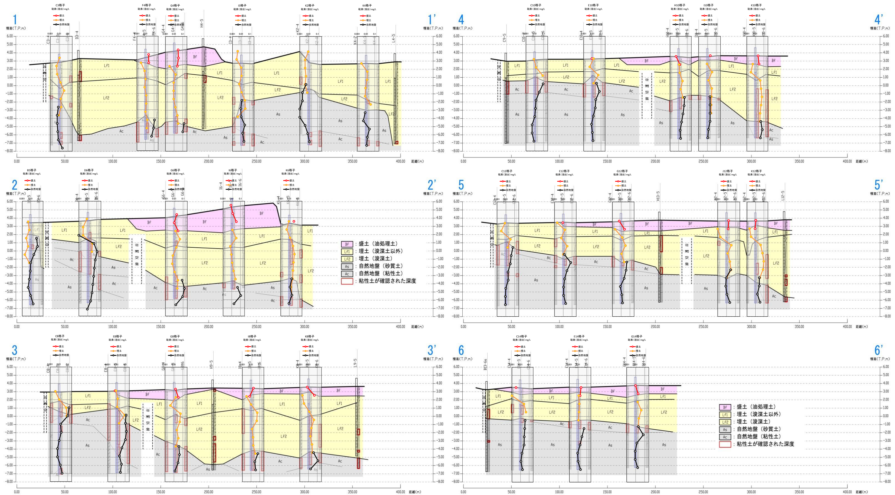
図 8.1.16 砒素土壌溶出量の深度別濃度分布状況と地質断面の重ね合わせ
