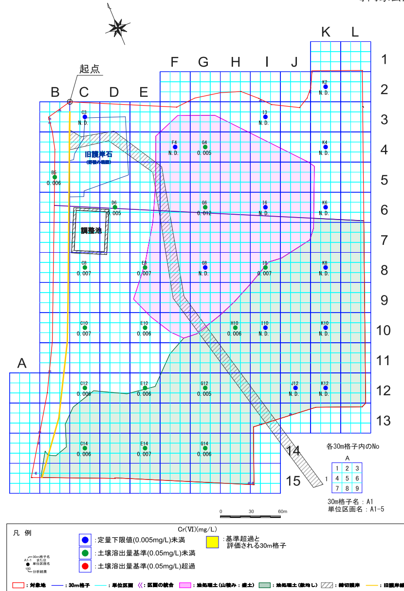
図 8.1.30 (2) 自然地盤における六価クロム土壤溶出量の平面分布
