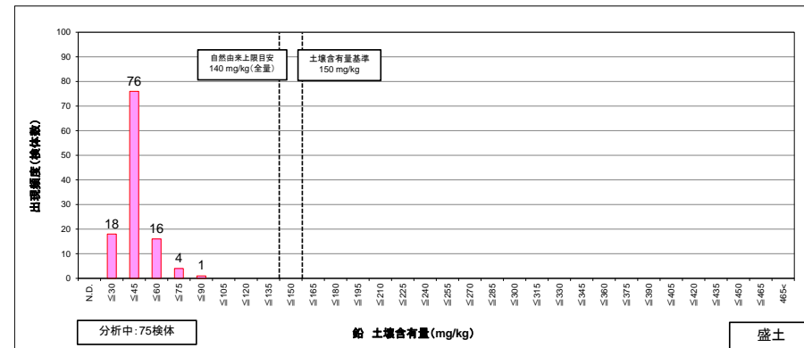
図 8.1.6 (1) 盛土における鉛土壌含有量の検出頻度分布
