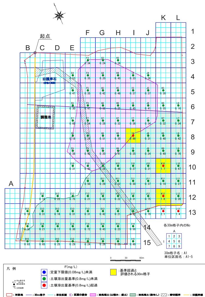
図 8.1.19 (1) 盛土におけるふっ素土壌溶出量の平面分布
