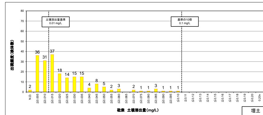
図 8.1.13 (2) 埋土における砒素土壤溶出量の検出頻度分布
