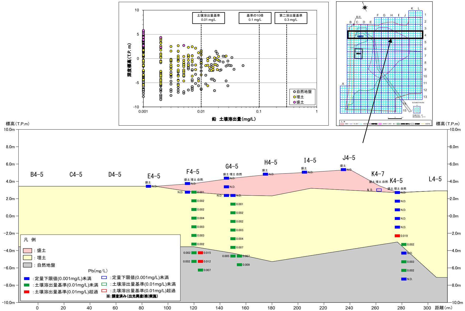
図 8.1.8 鉛土壤溶出量の深度別基準超過状況 (代表: 4 の 30m 格子行)
