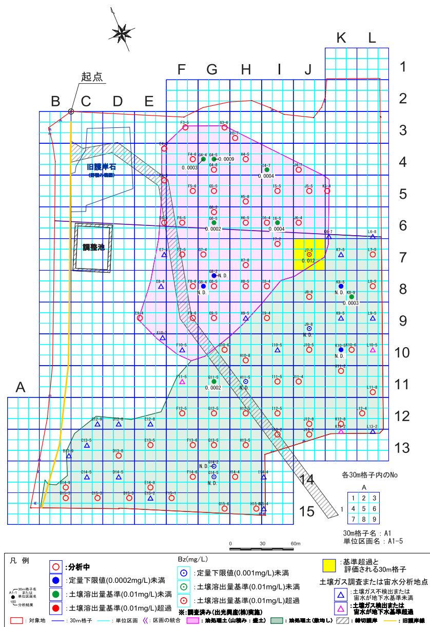
図 8.1.2 (2) 盛土におけるベンゼン土壌溶出量の平面分布 (盛土を対象とした深度別土壌調査結果)
