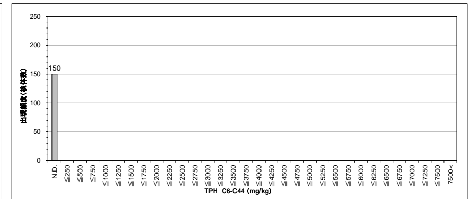
図 8.1.37 (3) 自然地盤における TPH (C6-C44) の検出頻度分布
