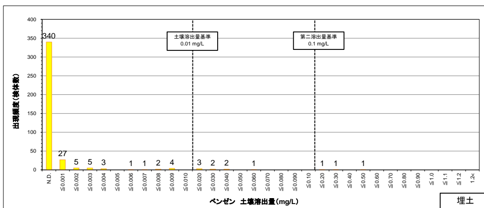
図 8.1.1 (2) 埋土におけるベンゼン土壌溶出量の検出頻度分布
