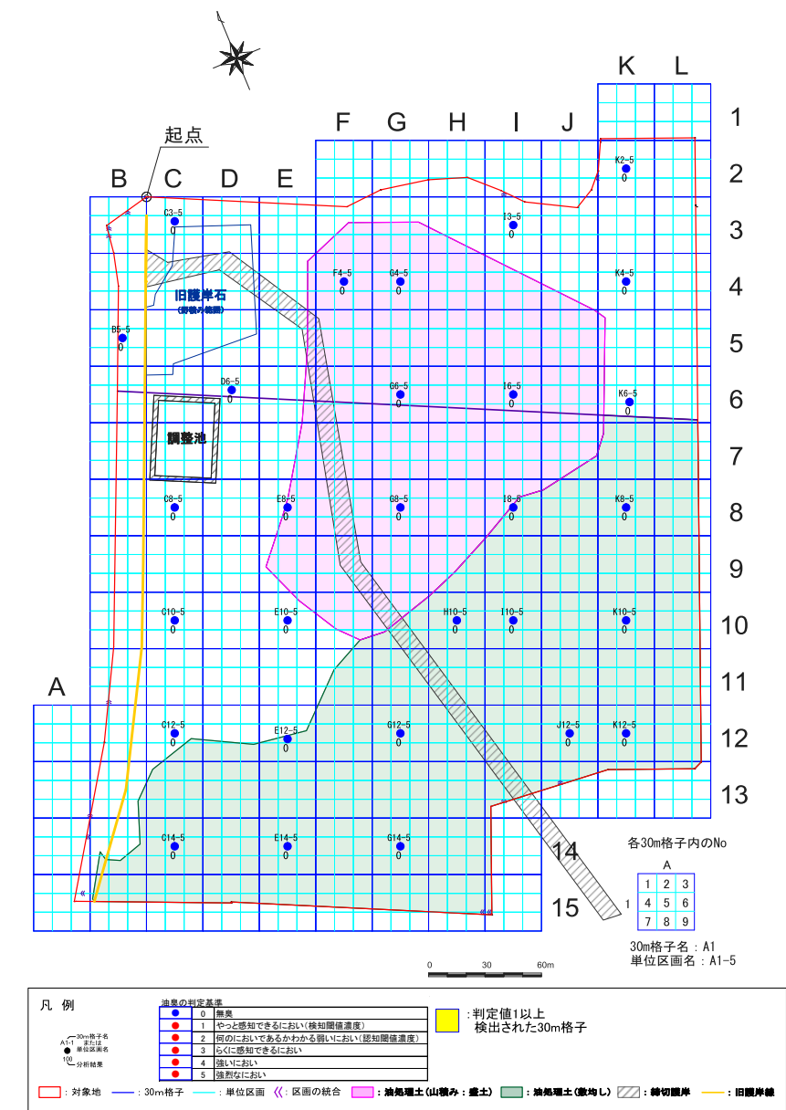
図 8.1.34 (3) 自然地盤における油臭の程度の平面分布
