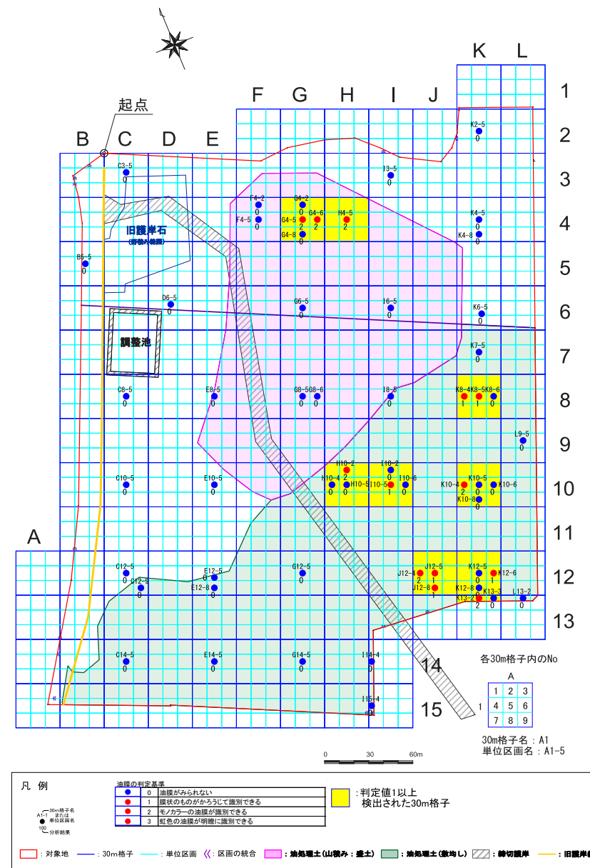
図 8.1.36 (2) 埋土における油膜の程度の平面分布
