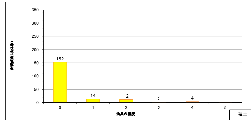
図 8.1.33 (2) 埋土における油臭の程度の検出頻度分布
