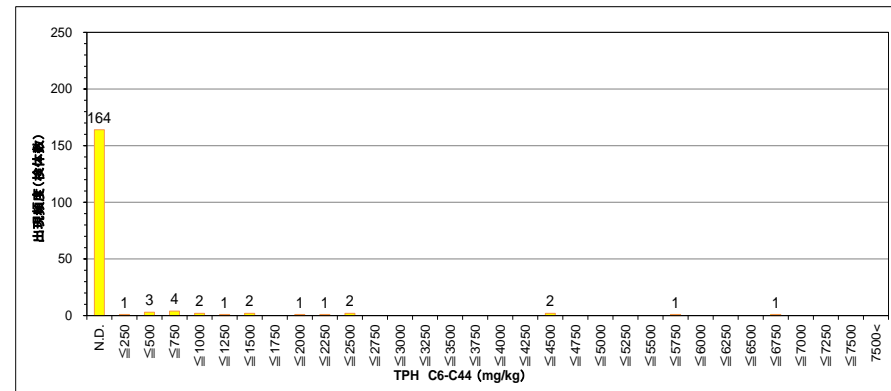
図 8.1.37 (2) 埋土における TPH (C6-C44) の検出頻度分布
