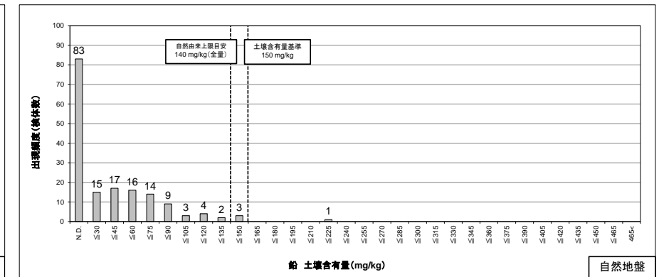
図 8.1.6 (3) 自然地盤における鉛土壌含有量の検出頻度分布
