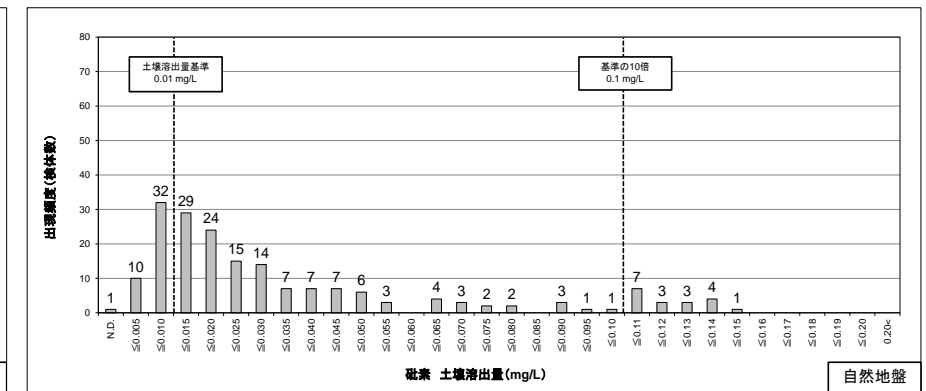
図 8.1.13 (3) 自然地盤における砒素土壤溶出量の検出頻度分布
