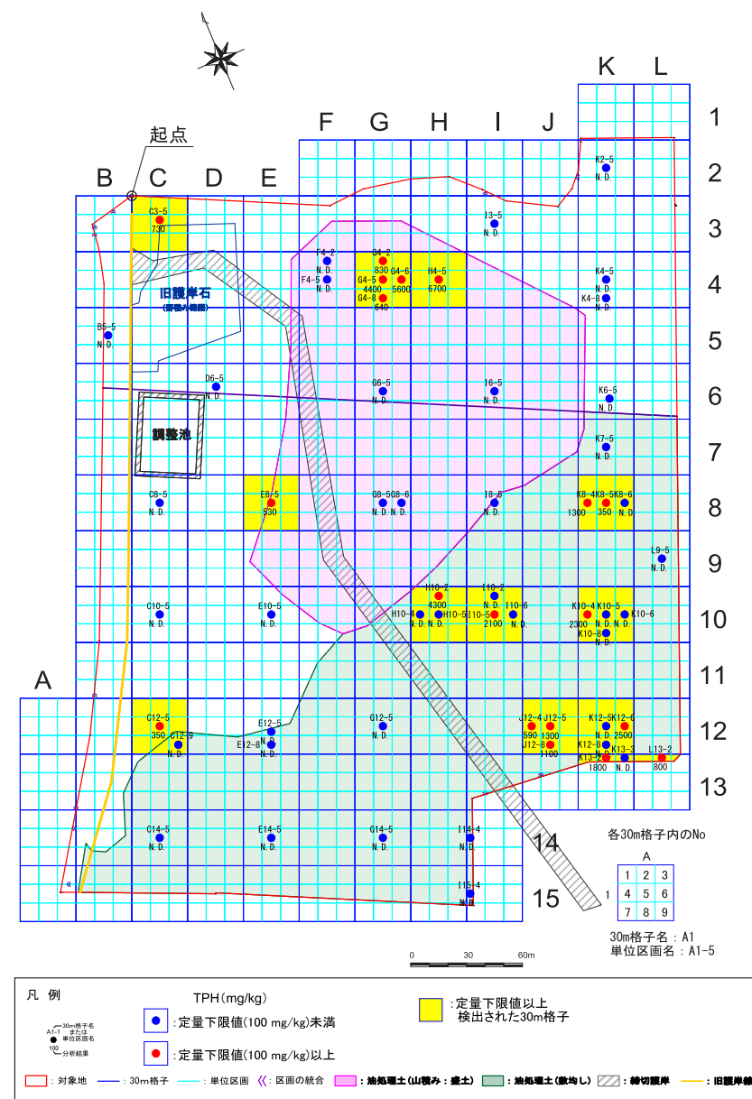
図 8.1.38 (2) 埋土における TPH (C6-C44) の平面分布
