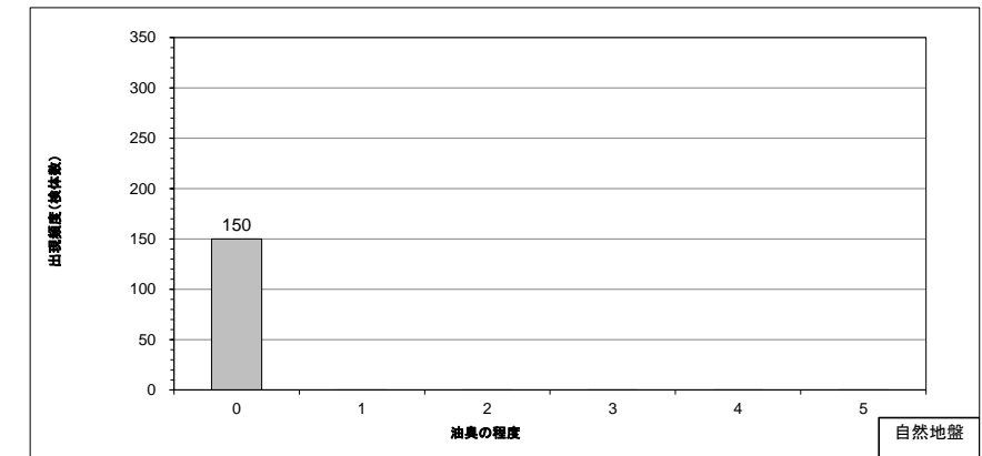
図 8.1.33 (3) 自然地盤における油臭の程度の検出頻度分布
