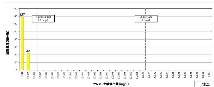
図 8.1.28 (1) 埋土におけるセレン土壌溶出量の検出頻度分布
