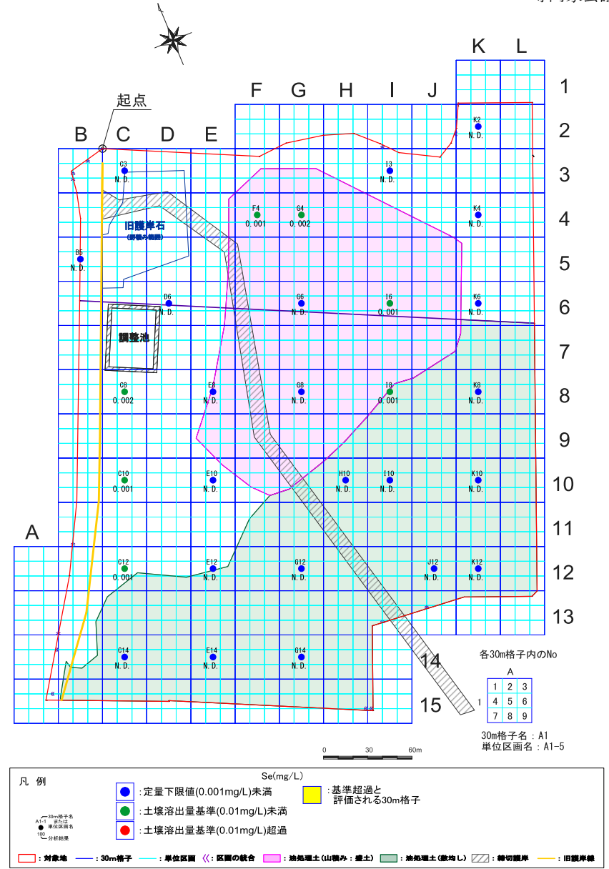
図 8.1.31 (2) 自然地盤におけるセレン土壌溶出量の平面分布
