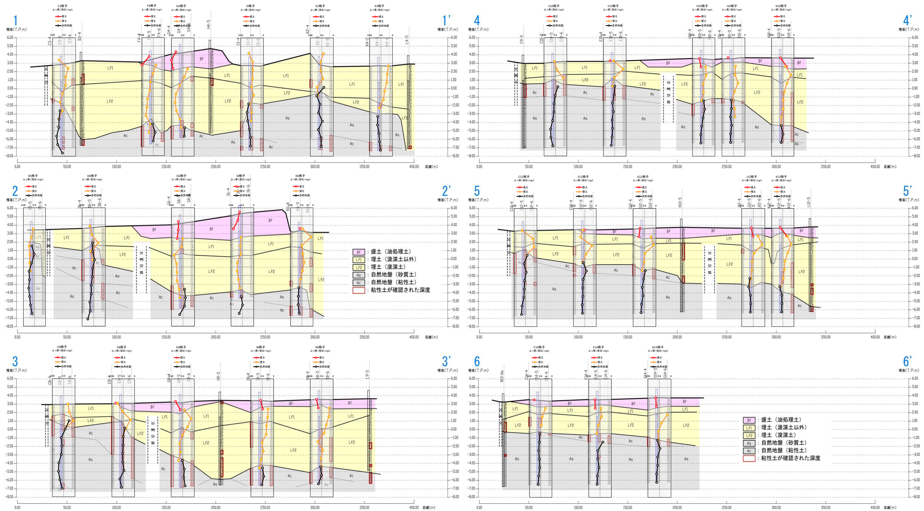
図 8.1.24 ふっ素土壌溶出量の深度別濃度分布状況と地質断面の重ね合わせ
