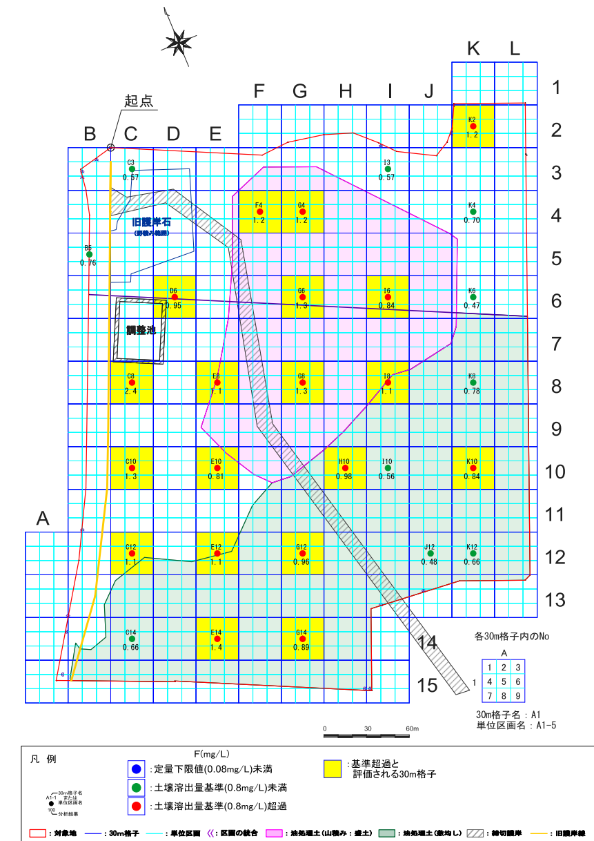
図 8.1.19 (3) 自然地盤におけるふっ素土壌溶出量の平面分布
