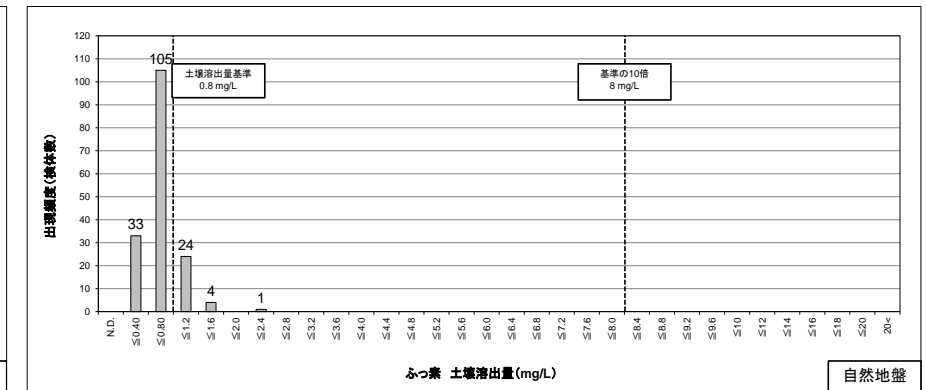
図 8.1.18 (3) 自然地盤におけるふっ素土壌溶出量の検出頻度分布
