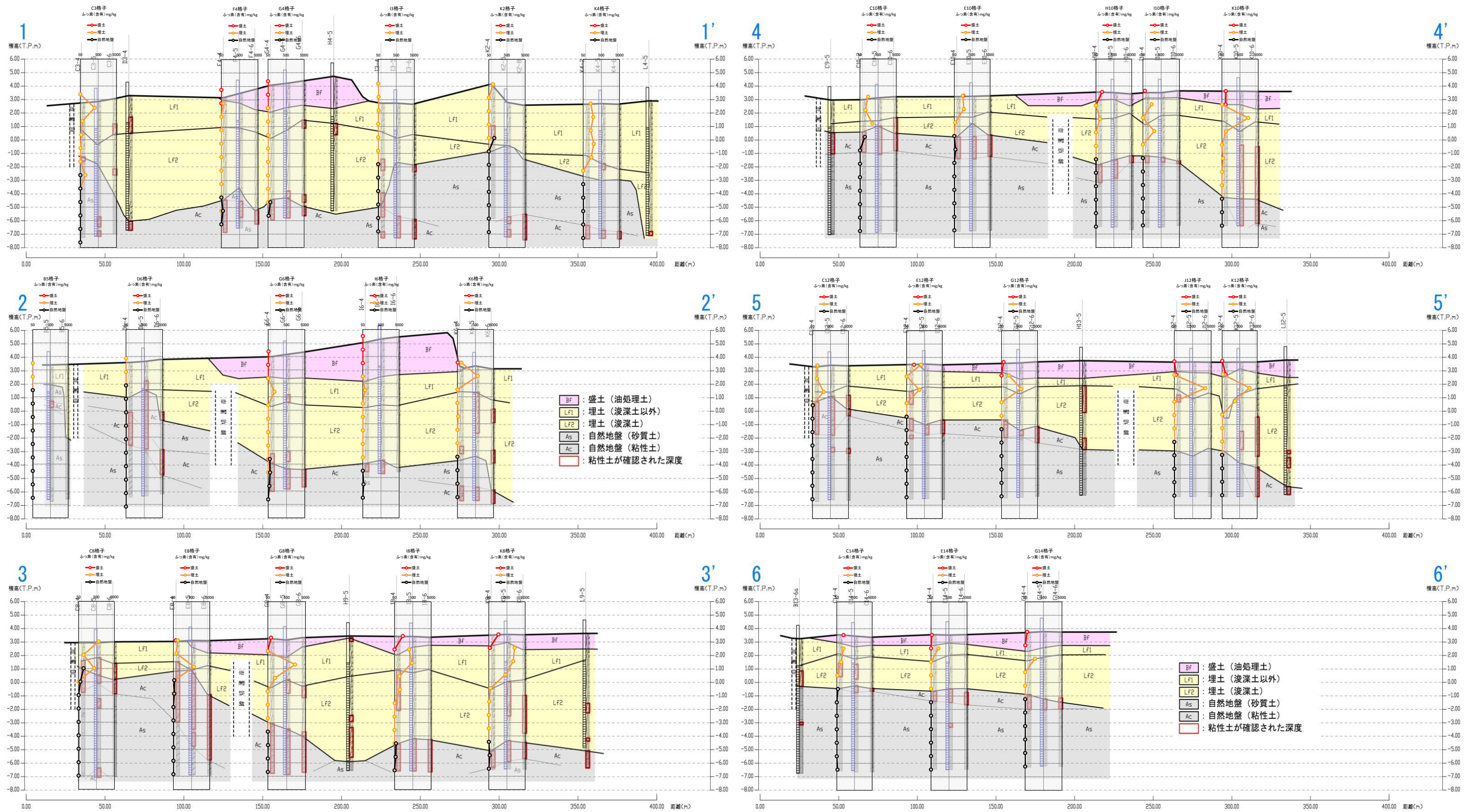
図 8.1.25 ふっ素土壌含有量の深度別濃度分布状況と地質断面の重ね合わせ
