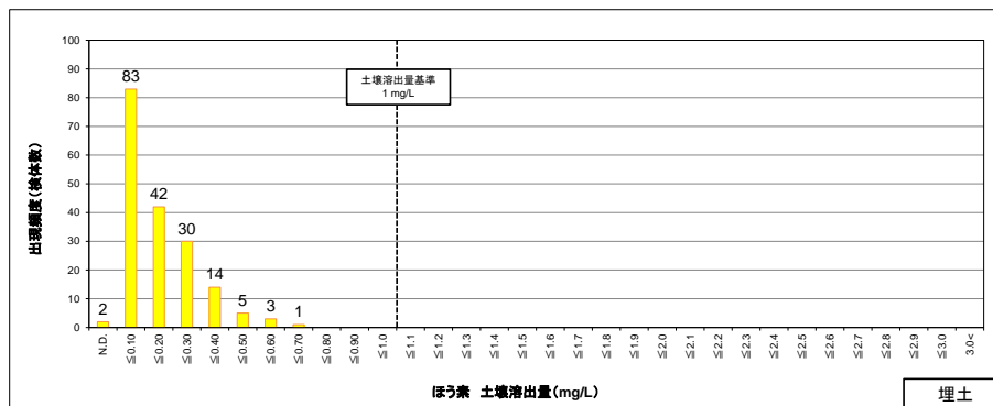
図 8.1.29 (1) 埋土におけるほう素土壌溶出量の検出頻度分布
