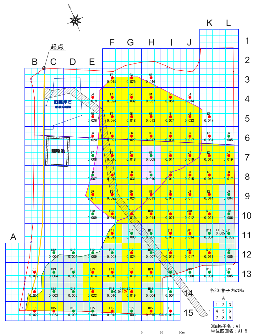
図 8.1.13 (1) 盛土における砒素土壤溶出量の検出頻度分布
