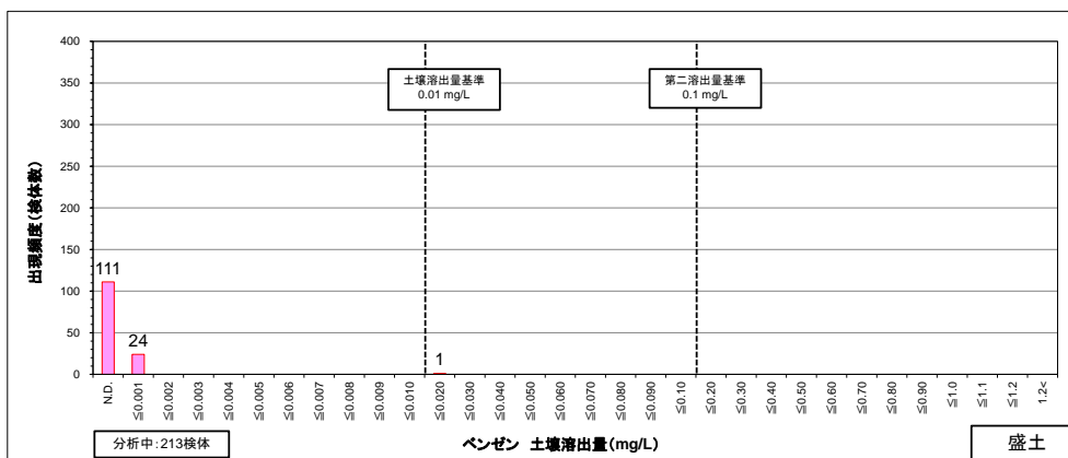
図 8.1.1 (1) 盛土におけるベンゼン土壌溶出量の検出頻度分布
