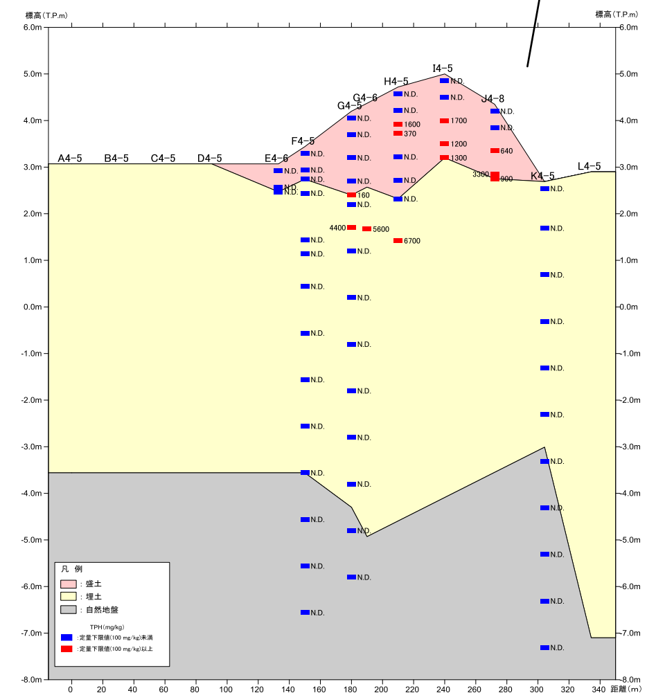
図 8.1.39 (3) TPH (C6-C44) の深度別基準超過状況 (代表：4 の 30m 格子行)
