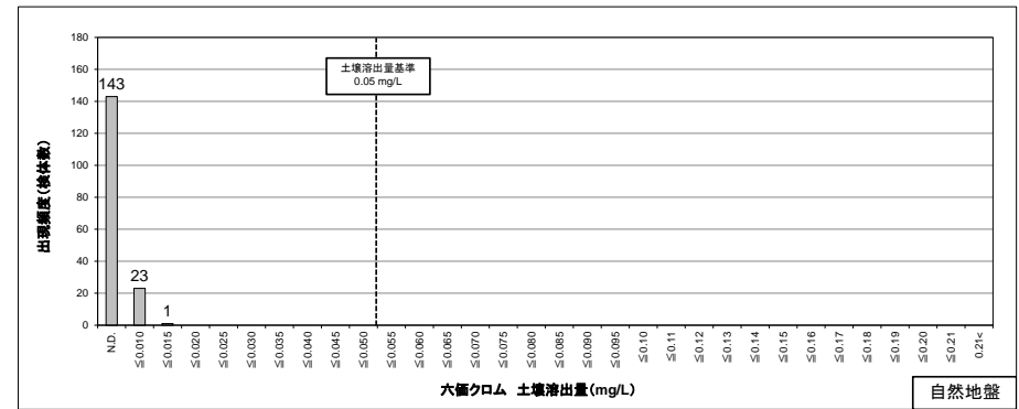
図 8.1.27 (2) 自然地盤における六価クロム土壌溶出量の検出頻度分布
