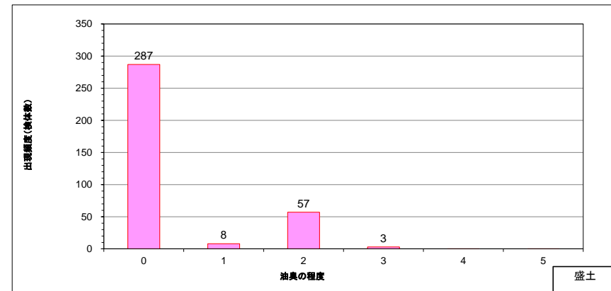
図 8.1.33 (1) 盛土における油臭の程度の検出頻度分布
