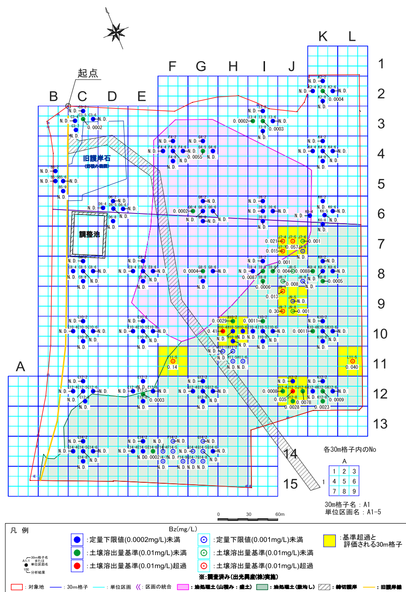
図 8.1.2 (3) 埋土におけるベンゼン土壌溶出量の平面分布
