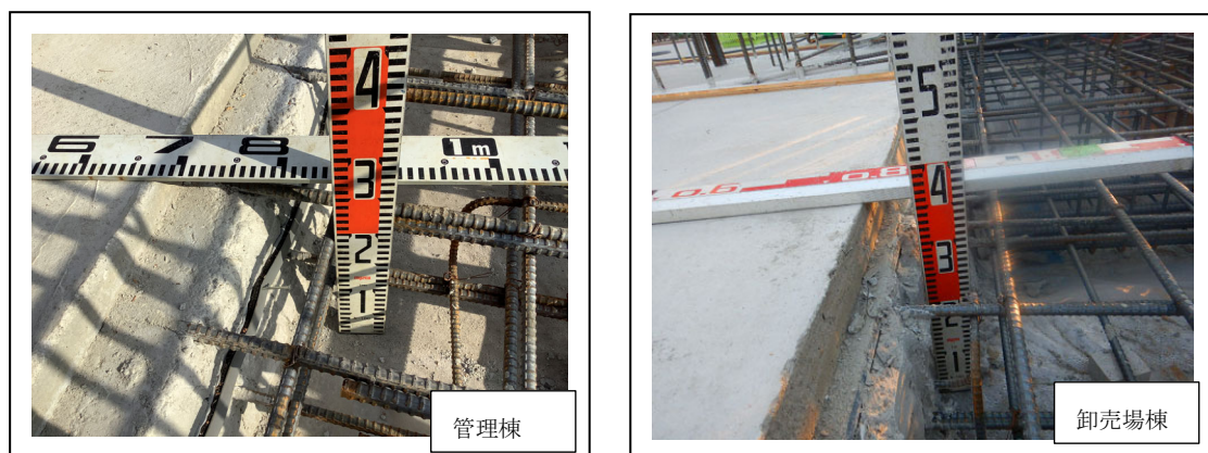
写真 2.2.6b 構造スラブの確認
