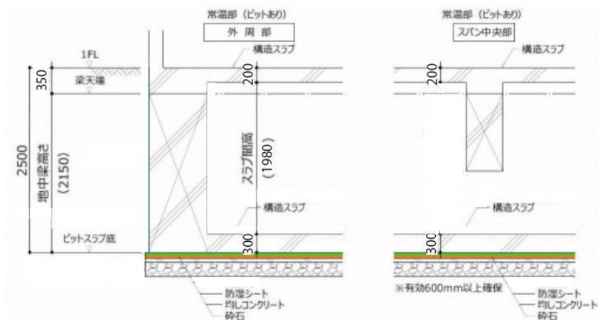
図 2.2.6a 構造スラブ（卸売場棟 1 階・配管ピットスラブ）
