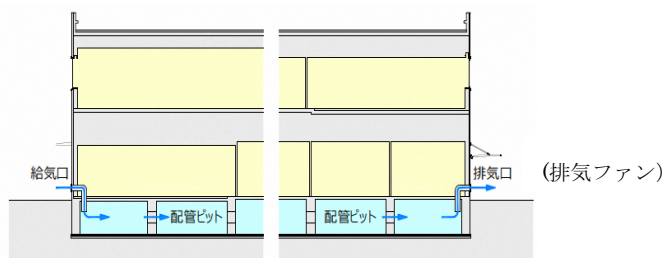
図 2.2.11a 第 3 種換気方式のイメージ図
