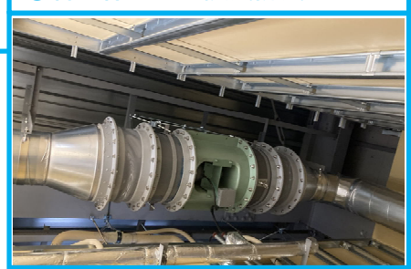
⑥管理棟ピット換気排気ファン
