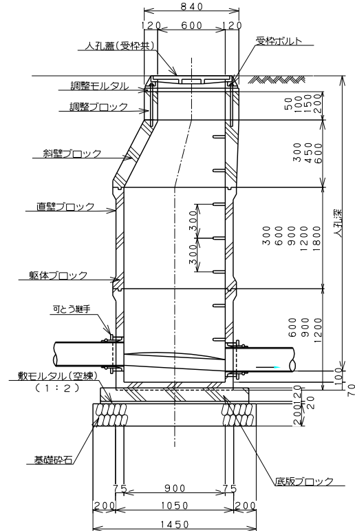
B-B 断面図
