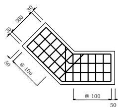
U型側溝45度折れ点部分詳細図
