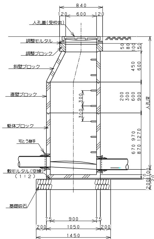
A-A 断面図
