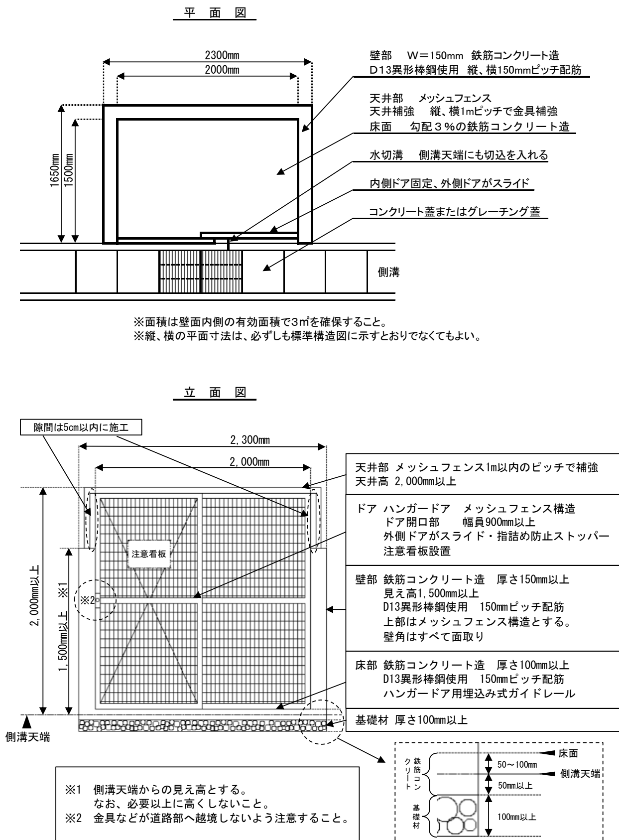
(図50)ごみ収集場標準構造図
