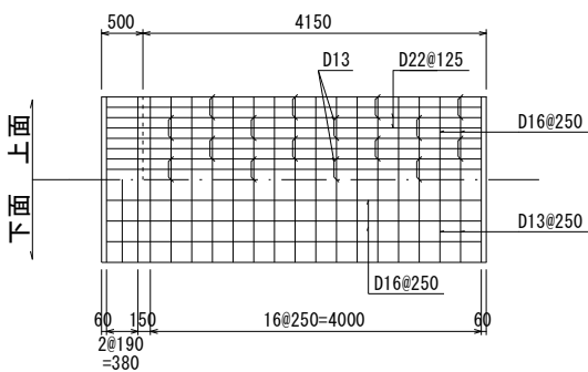
底版配筋図
