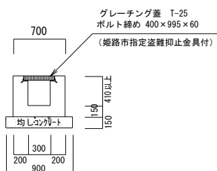
A—A' 断面图
