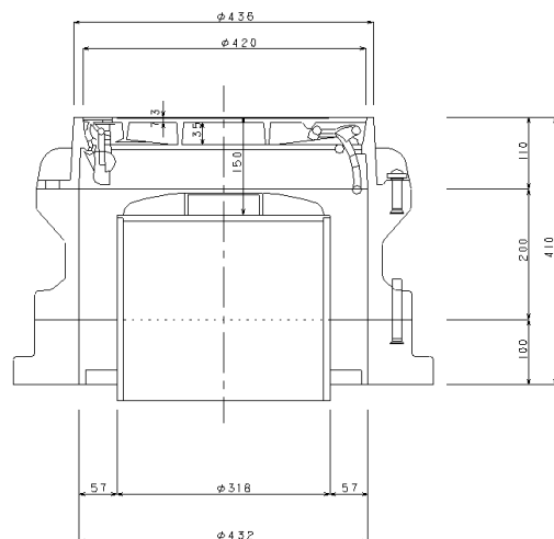
断面図(拡大)
