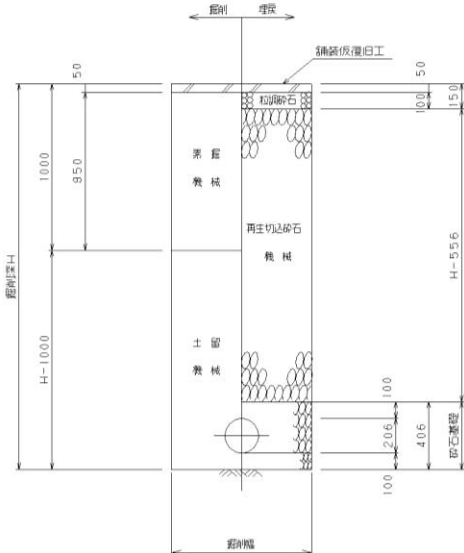
PRPφ200(土留あり)
