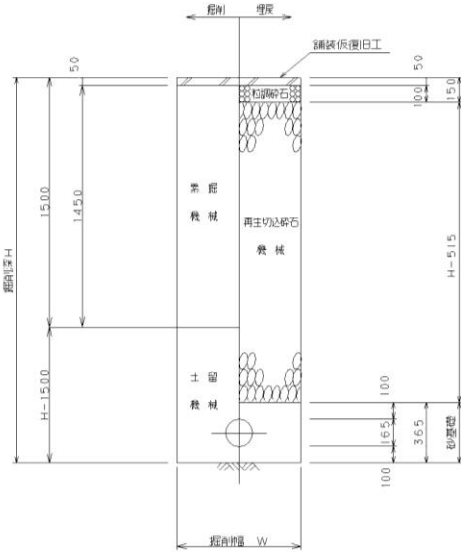
取付管VUφ150
