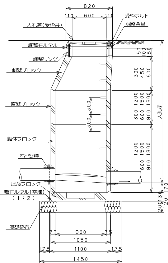
B-B 断面图
