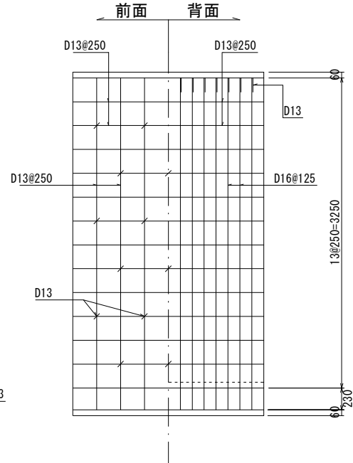
縦壁配筋図
