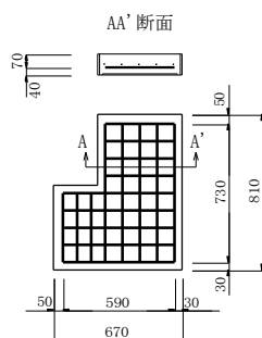
U型側溝90度折れ点部分詳細図
