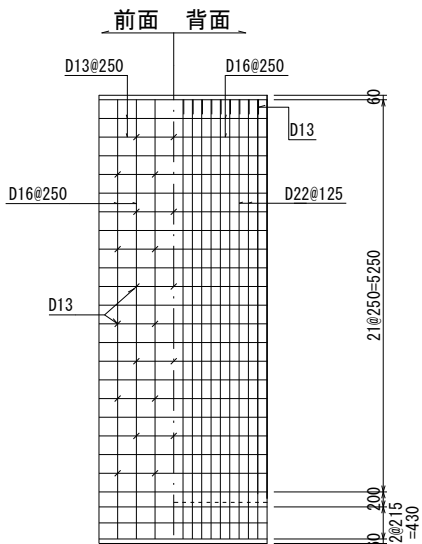
縦壁配筋図
