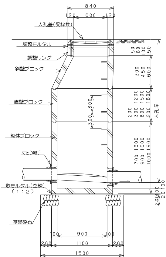
A-A 断面图
