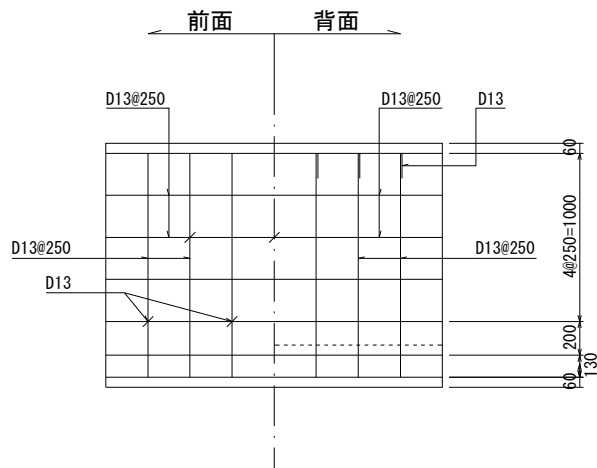
縦壁配筋図
