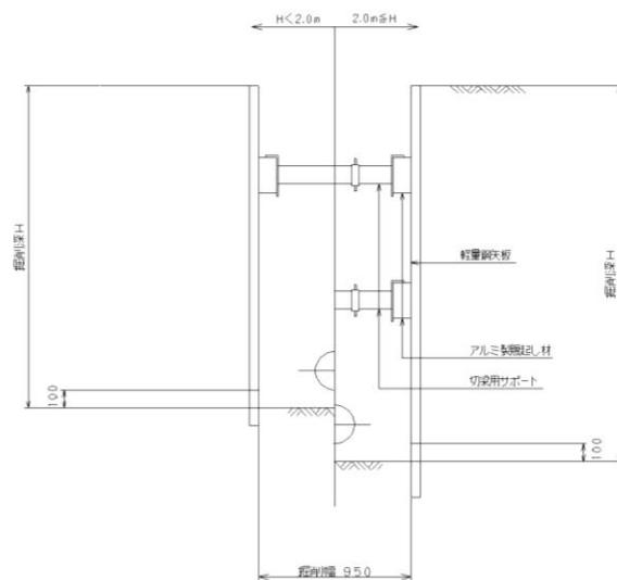
軽量鋼矢板 (掘削深 H=1.5 m 超)
