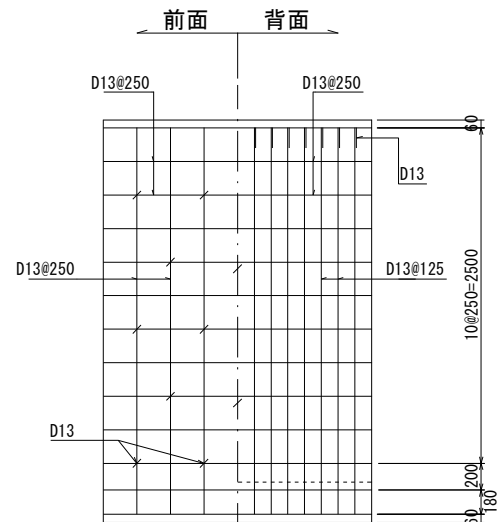
縦壁配筋図
