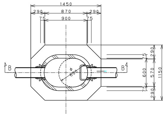
平面図
