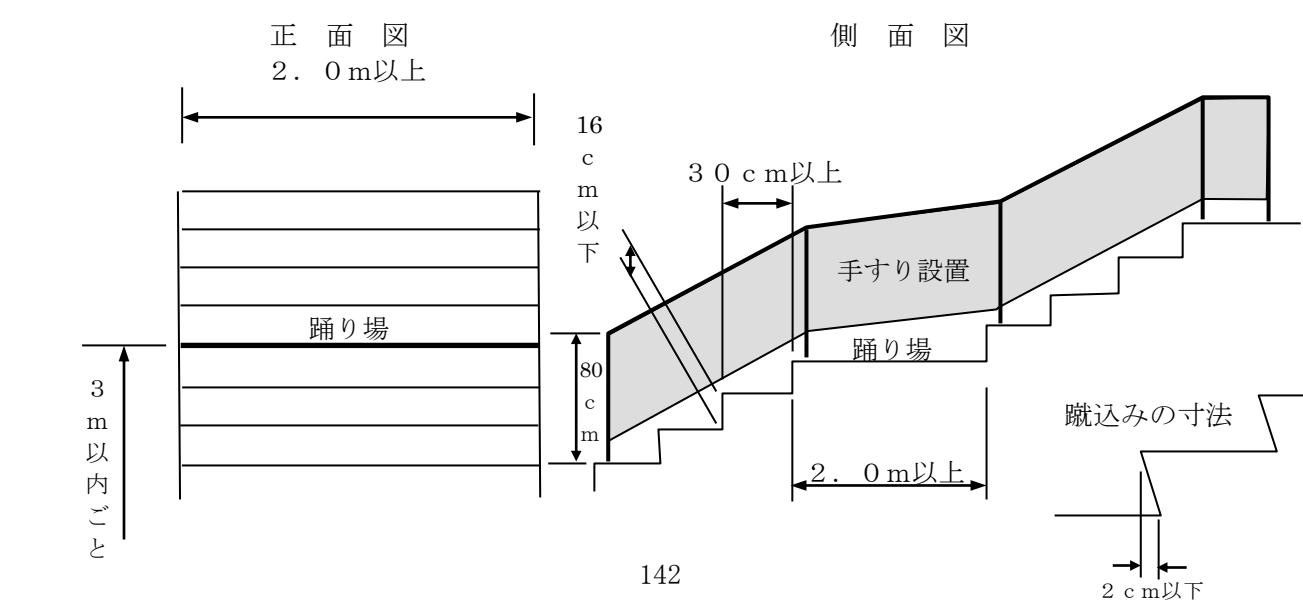
(図 18) 階段標準図
