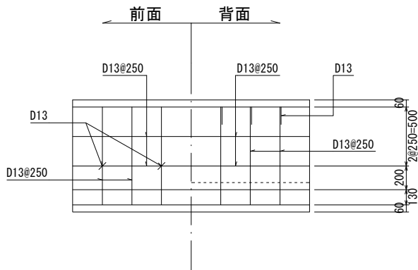
縦壁配筋図
