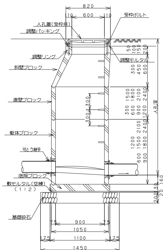
E-E 断面图
