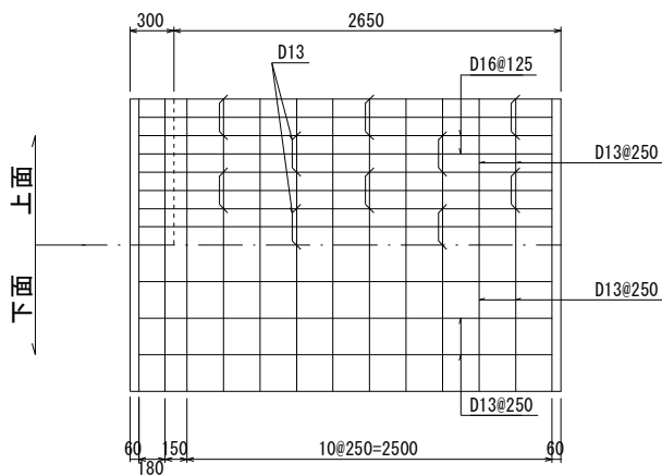
底版配筋図
