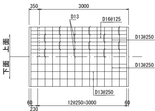
底板配筋図
