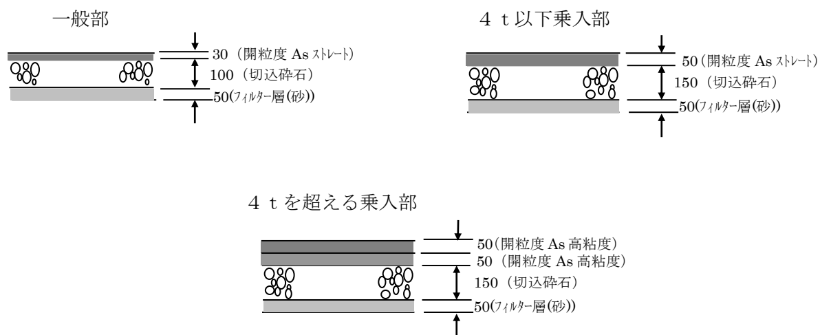
開粒度アスファルトコンクリート舗装（13）標準図
