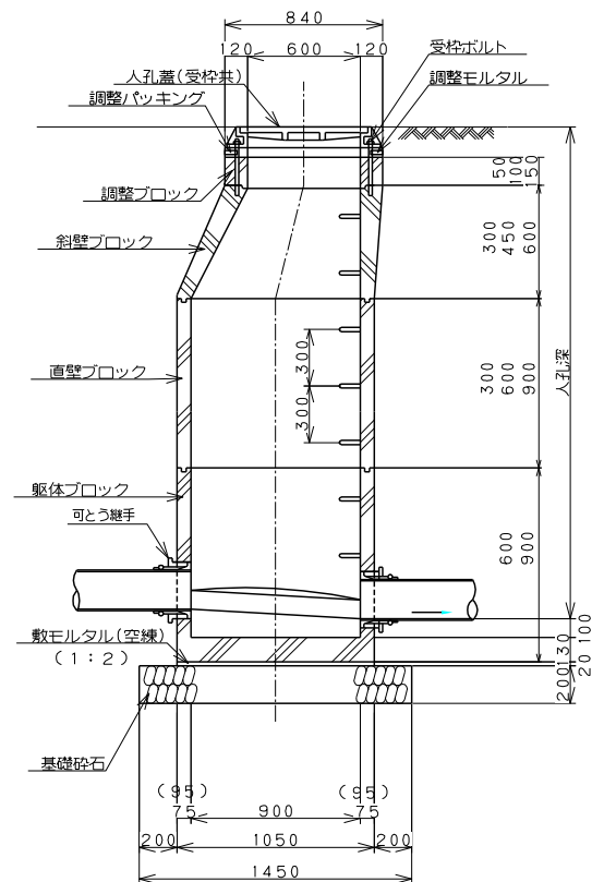
C-C 断面図
