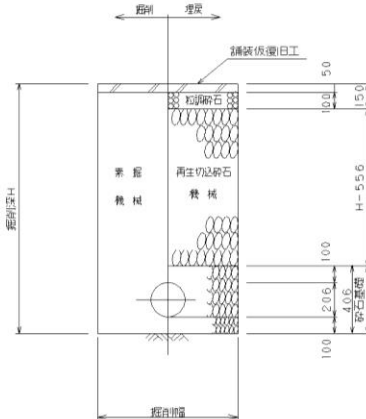
PRP \phi 200(素掘)
