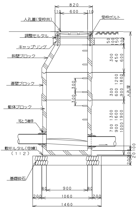
D-D 断面図
