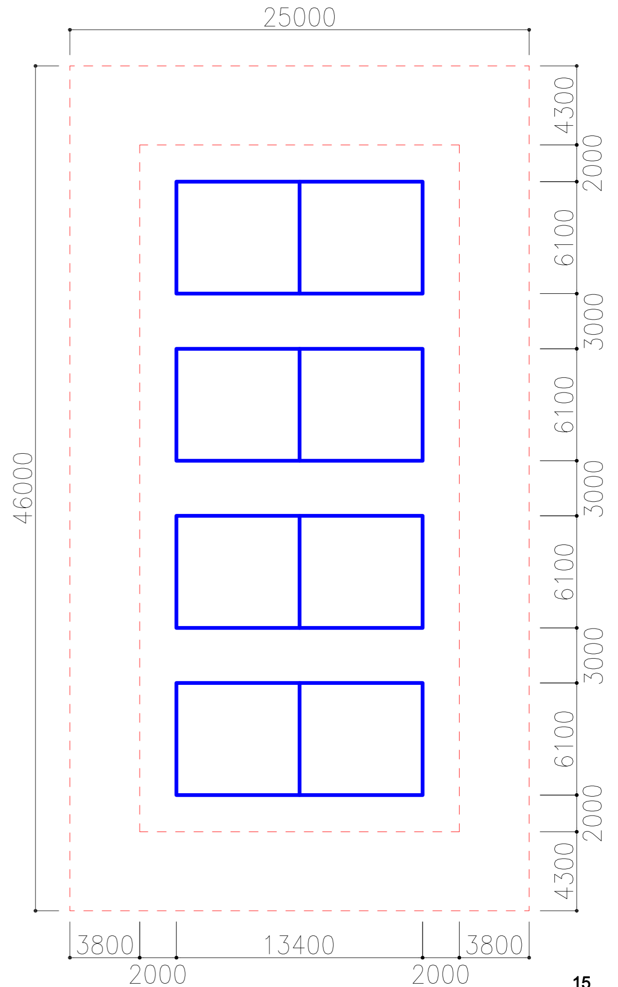
サブアリーナ（バドミントンコート4面）
