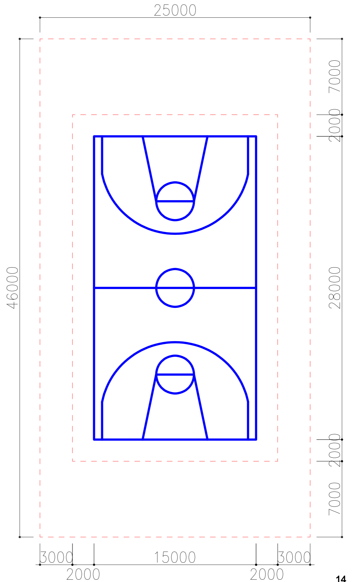
サブアリーナ（バスケットボールコート1面）
