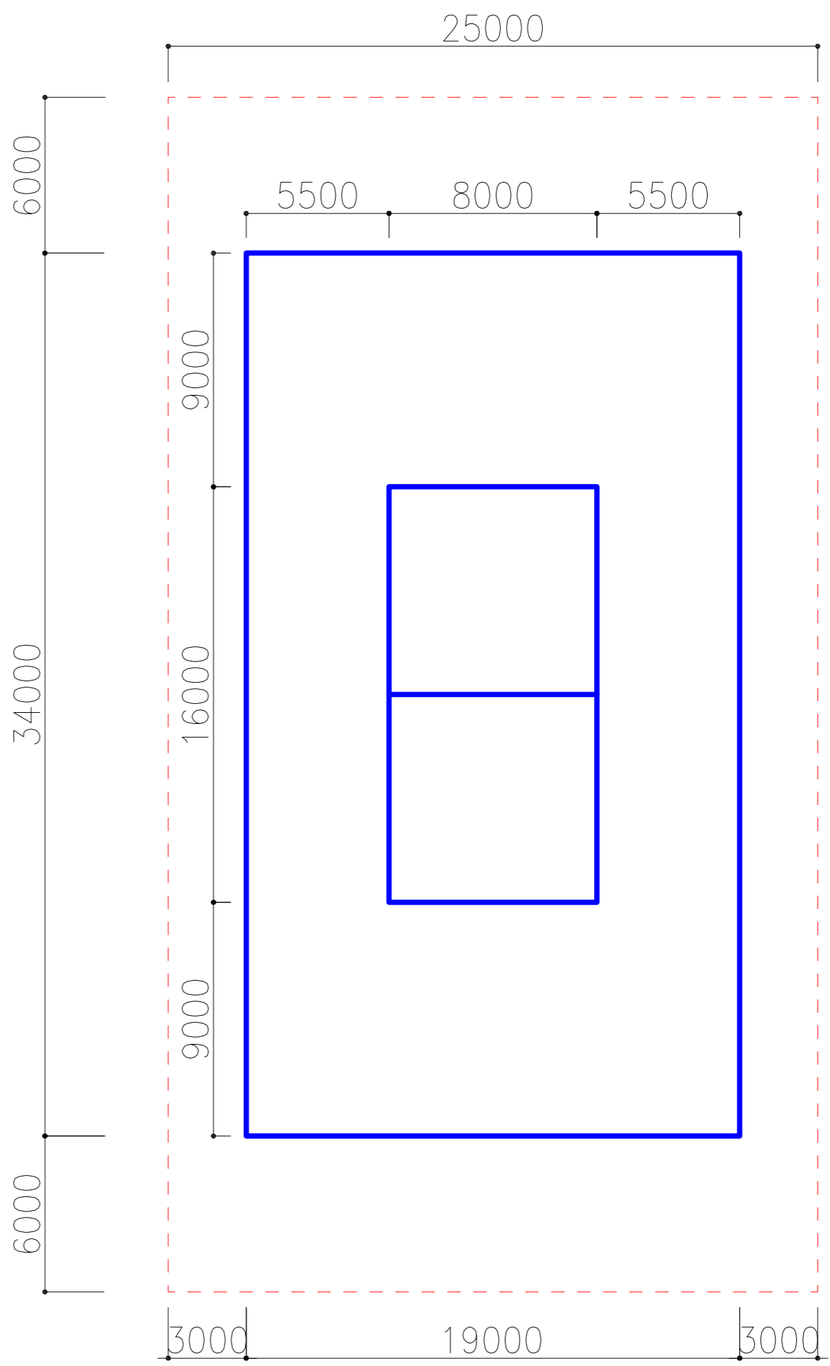
サブアリーナ（小学生 バレーボールコート1面）
