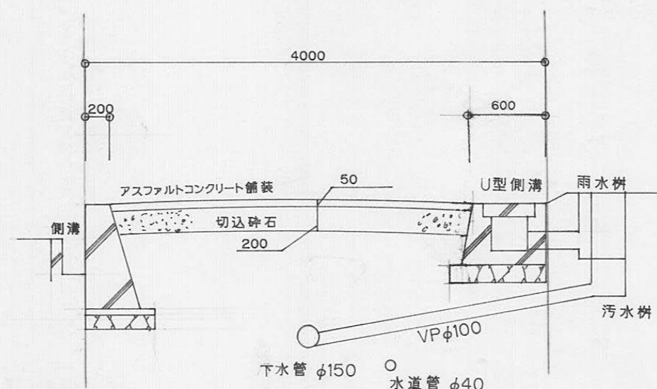
道路構造図 S=1/50
