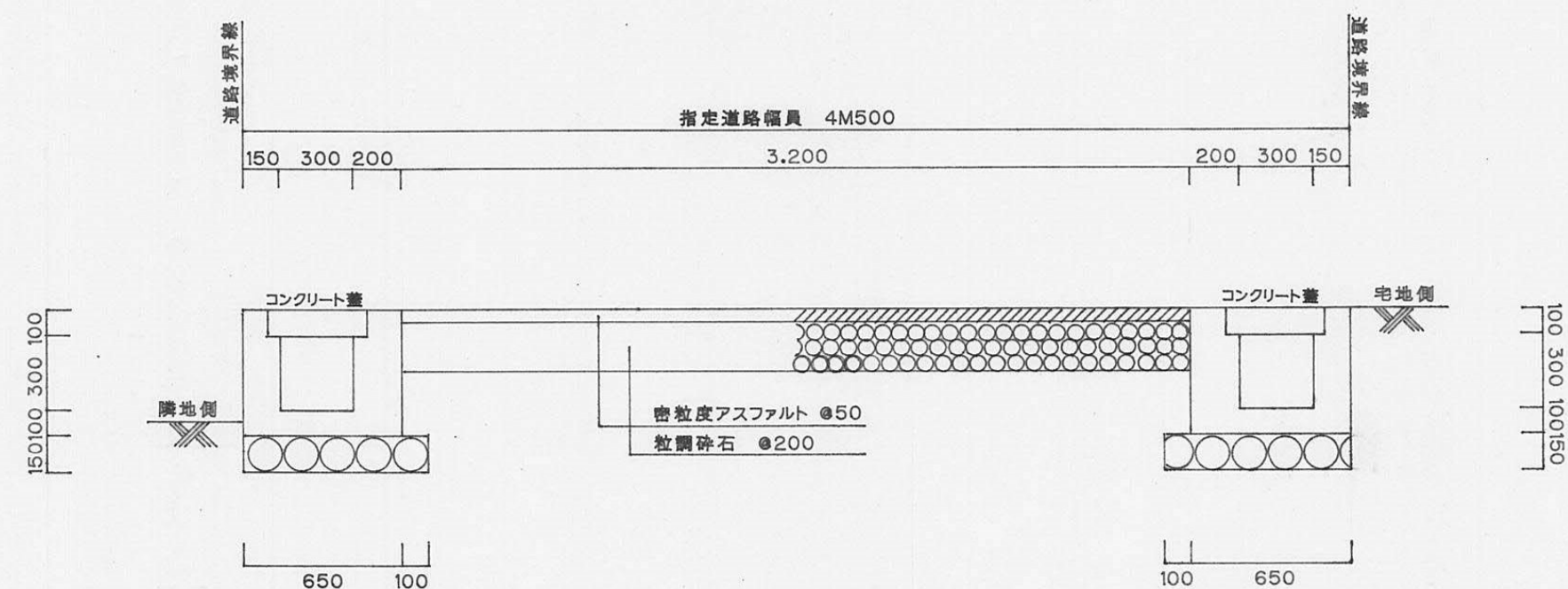
横断・構造図 S=1/30
