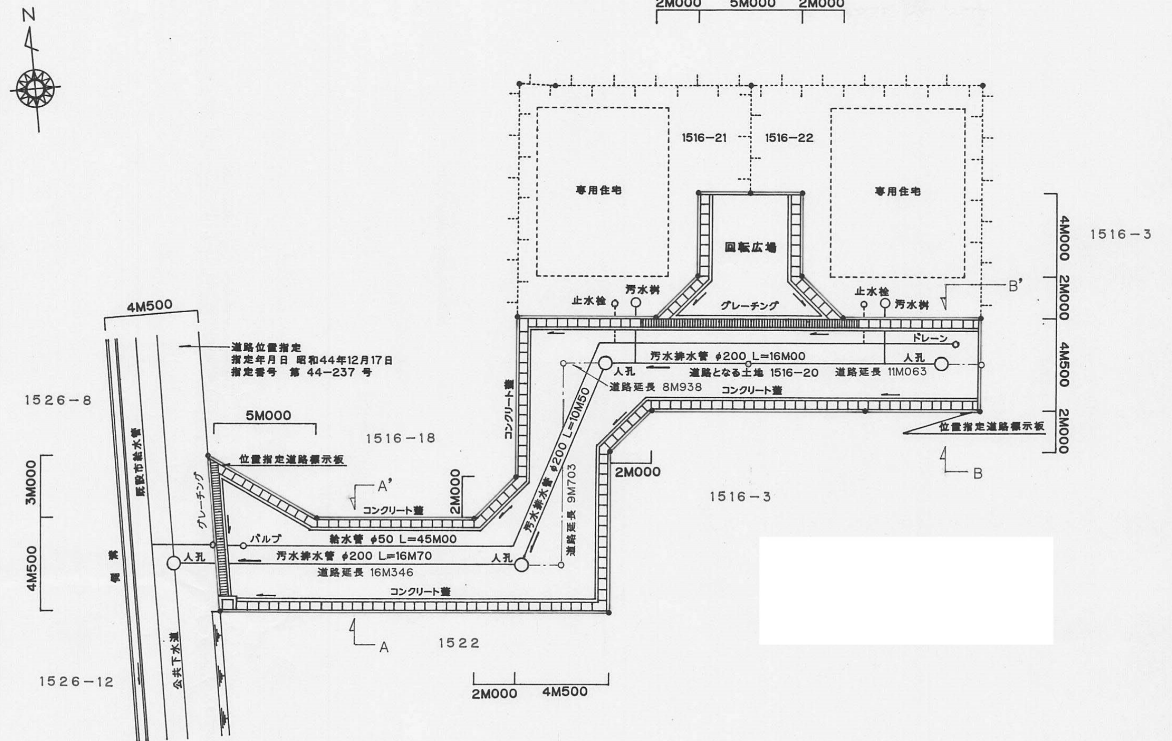
平面图 S=1/200
