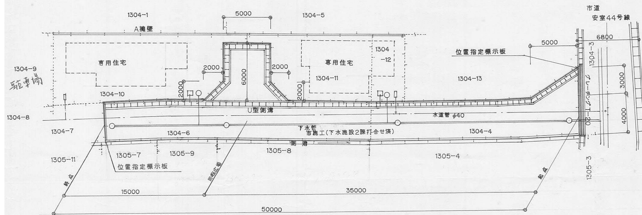
造成計画平面図 S=1/250
