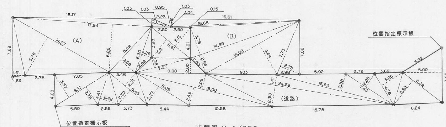
求積図 S=1/250
