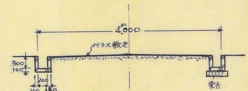
断面図 1/50 A 15
