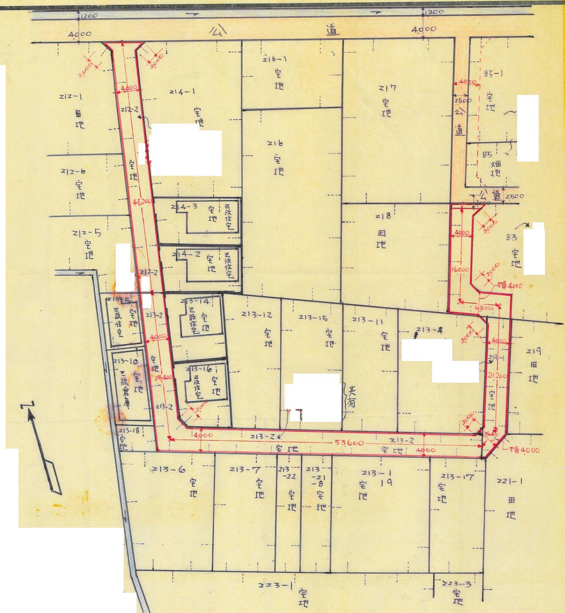
平面配置図 1/400.
