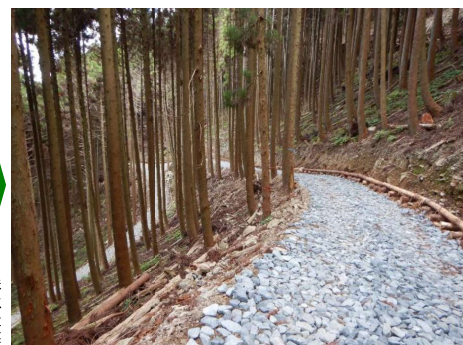
<市有林内に開設した作業道（安富町地内）>
