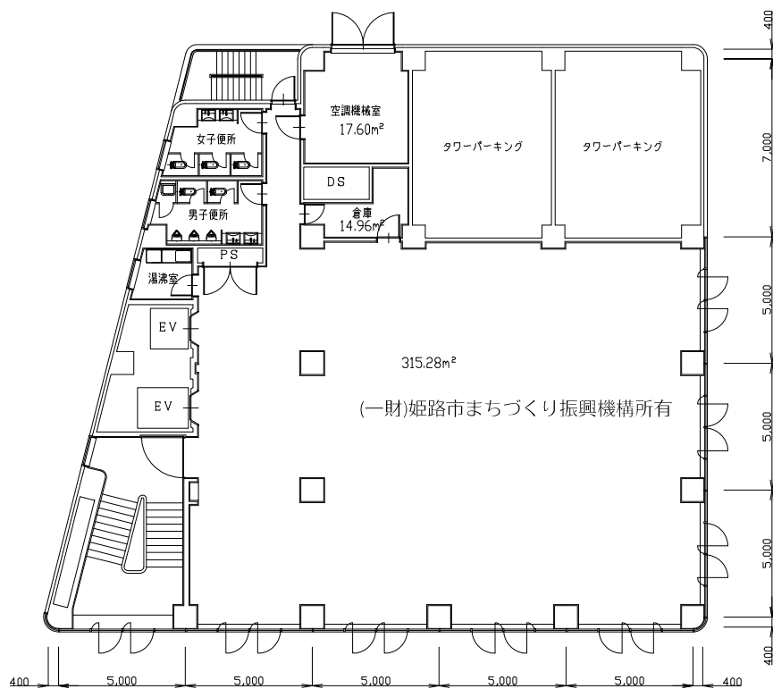
8階平面図
