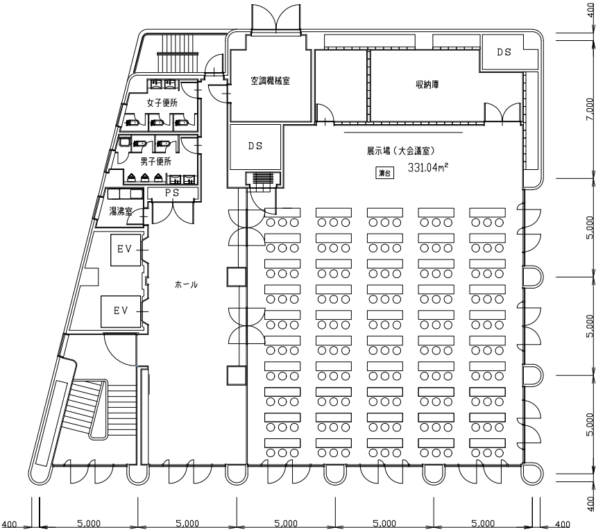
9階平面図
