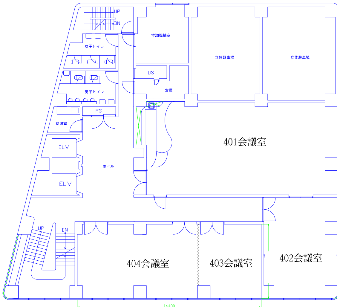
4階平面図
