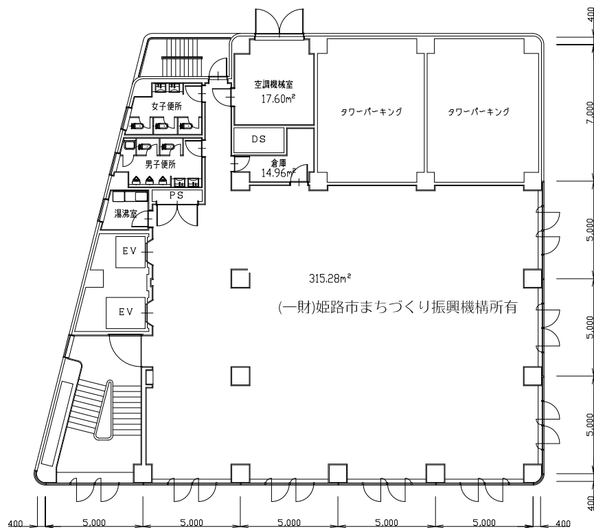
7階平面図
