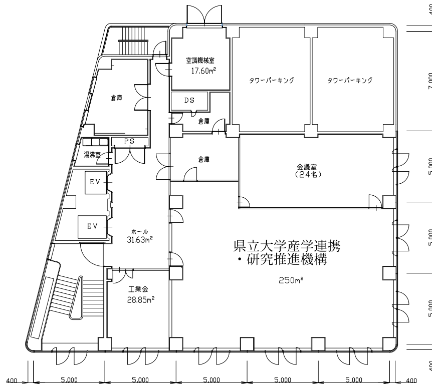
3階平面図
