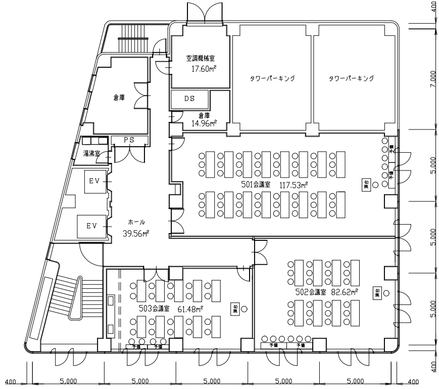
5階平面図
