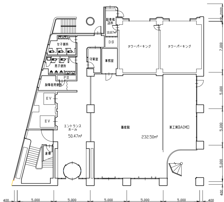
1 階平面図
