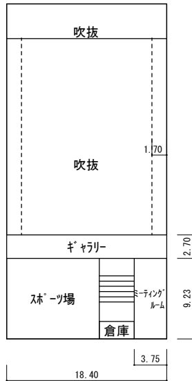
屋内運動場
