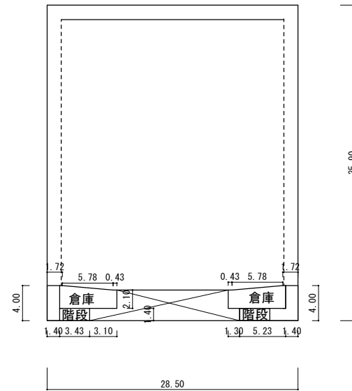
2階 平面図
