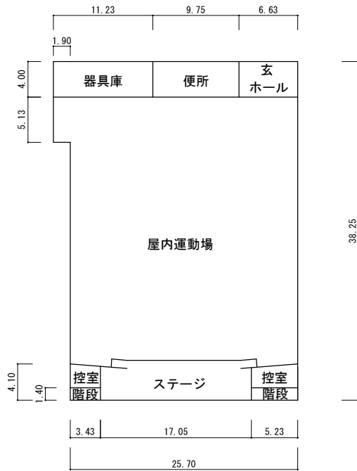
1階 平面図
