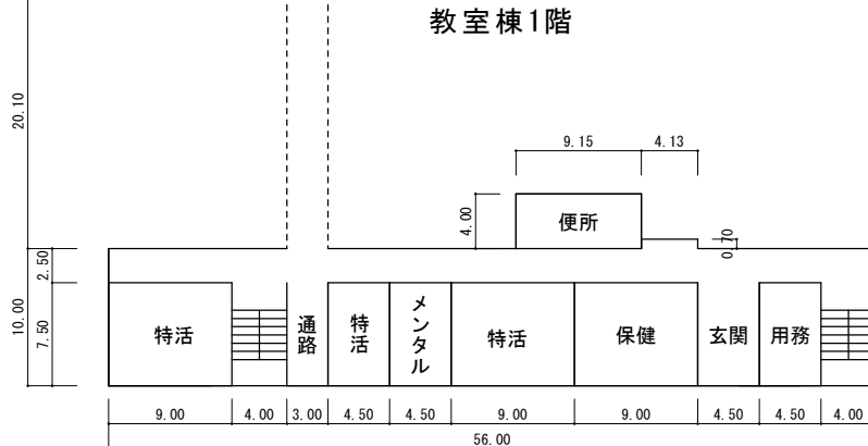
管理教室棟
