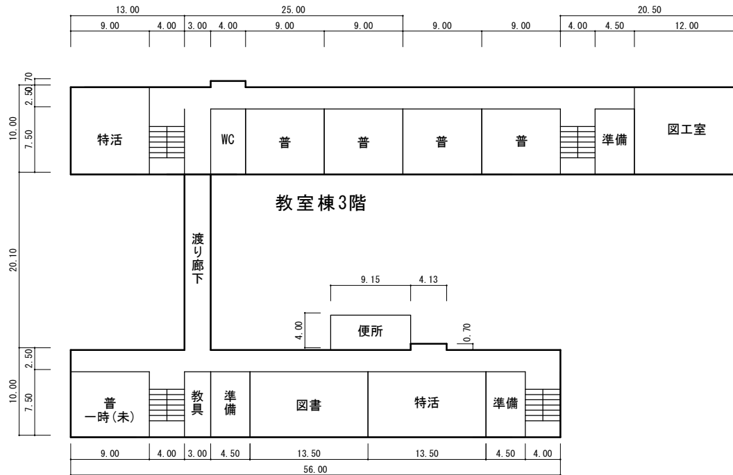
3階 平面図
