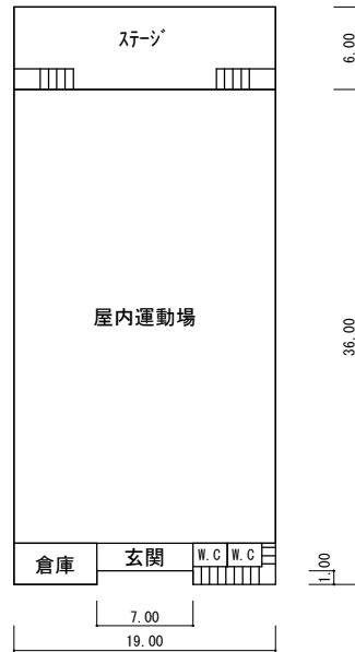
1階
