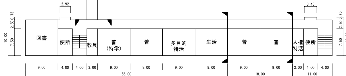
教室棟2階
