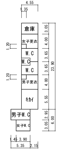
屋外便所
