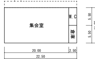
2F
