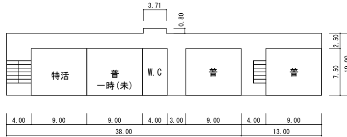
教室棟1階
