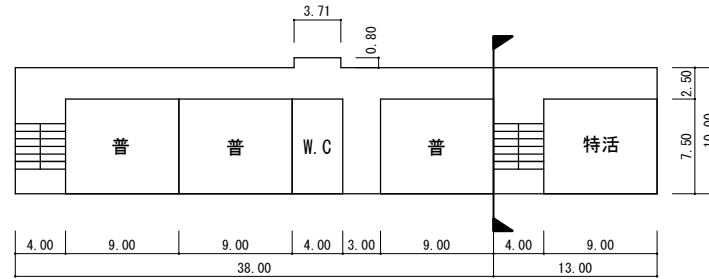
教室棟 2階
