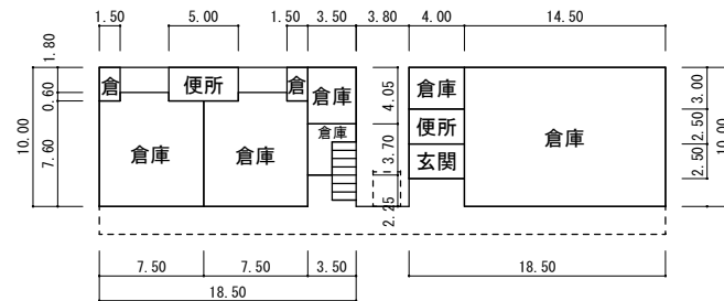
1階平面図
