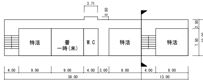
教室棟 3階
