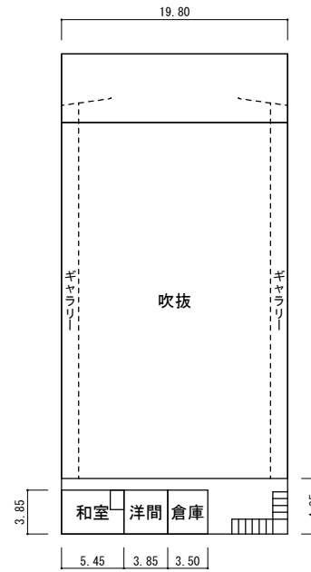
2階
