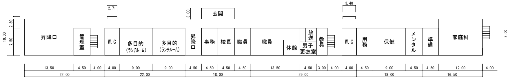
四郷学院前期課程校舎平面図
