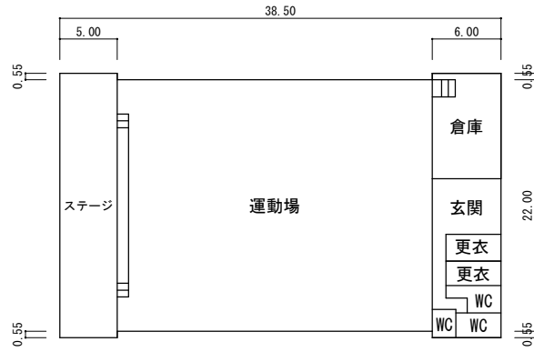
1 階
