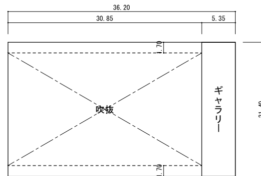
2階
