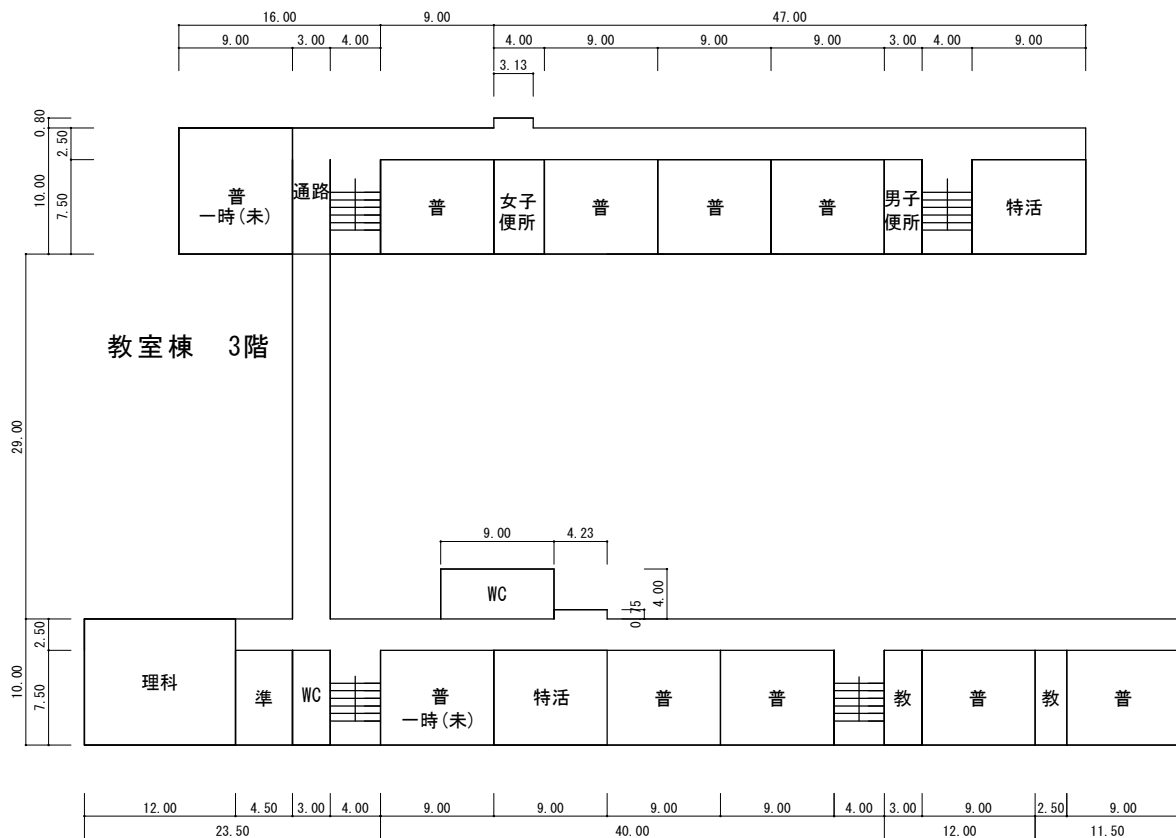
教室棟 3階
