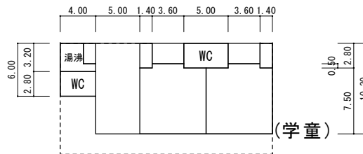
1階平面図
