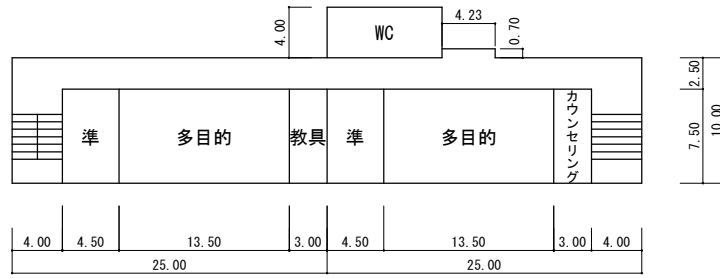
管理棟 3階
