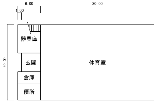
1階
