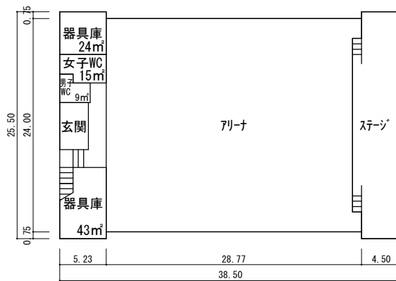
屋内運動場
