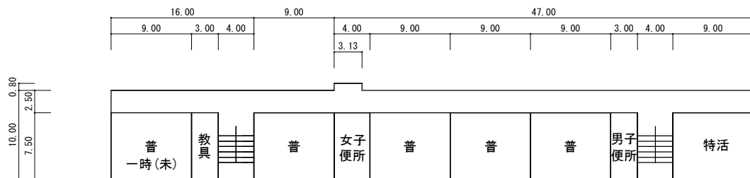
教室棟 4階
