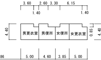
附属室
