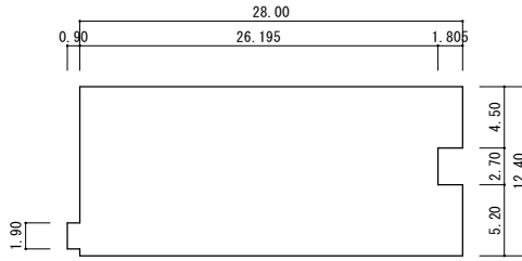
給食室 1階
