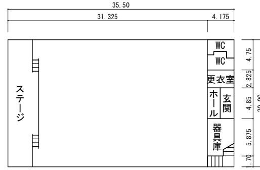
1階
