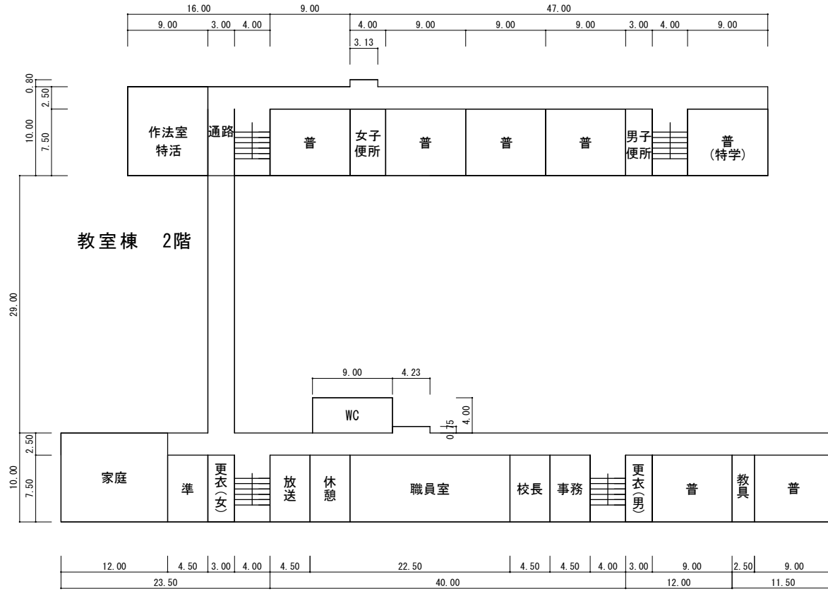
教室棟 2階
