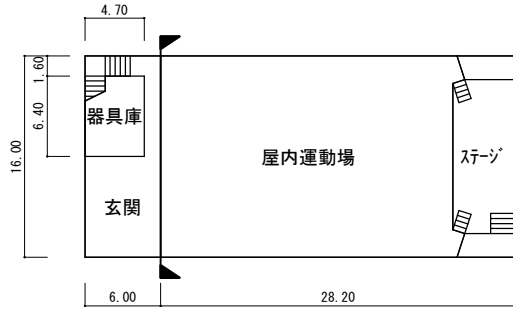
1階
