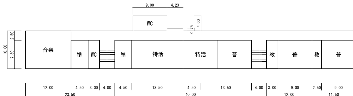
教室棟 4階
