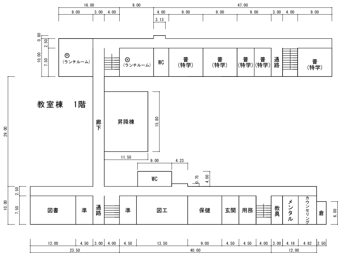
教室棟1階
