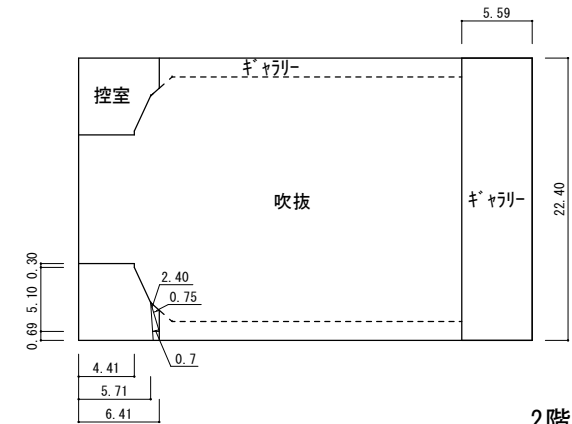
2階
