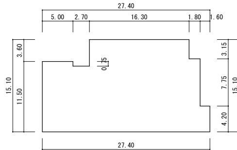
給食室
